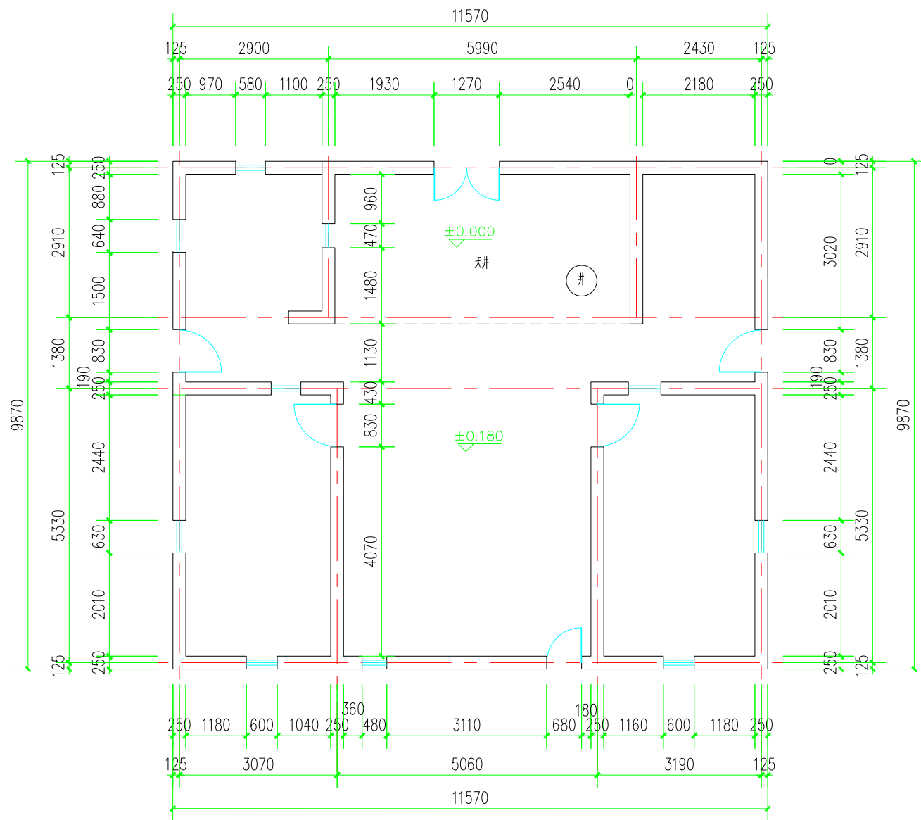
一层平面
