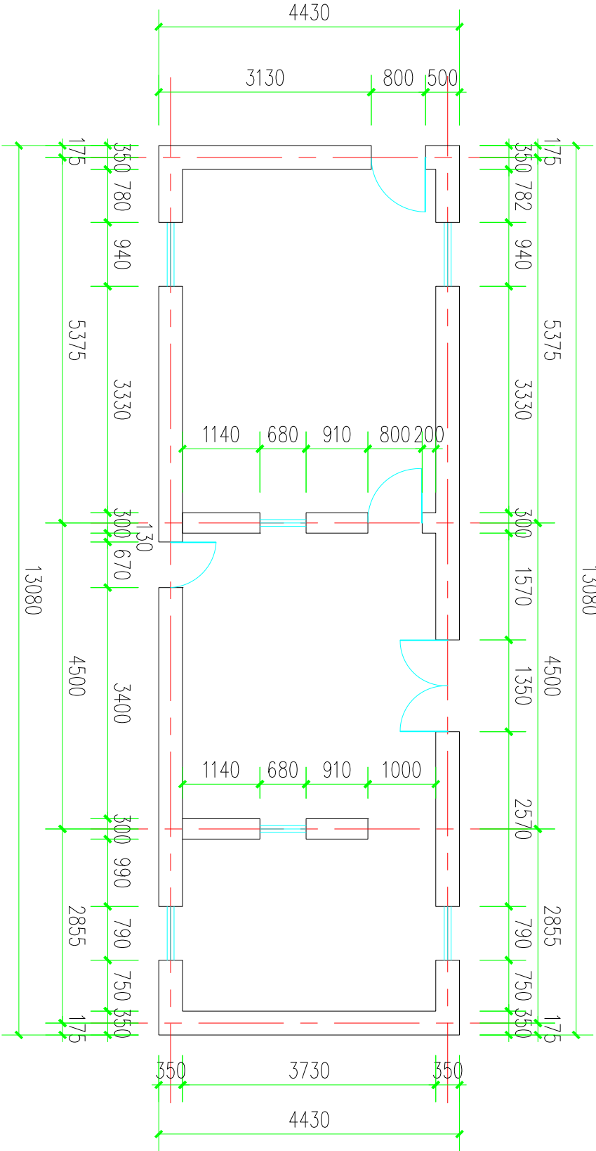
一层平面
