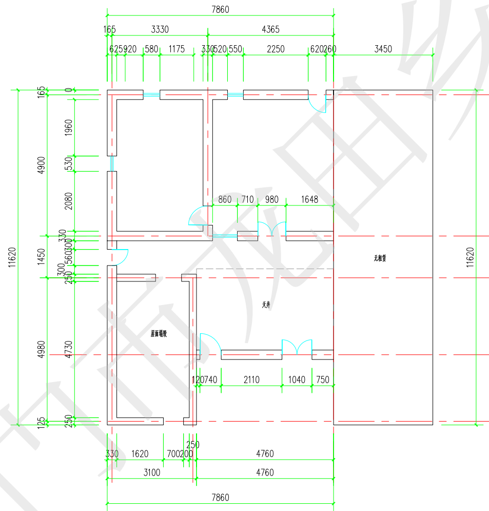
一层平面
