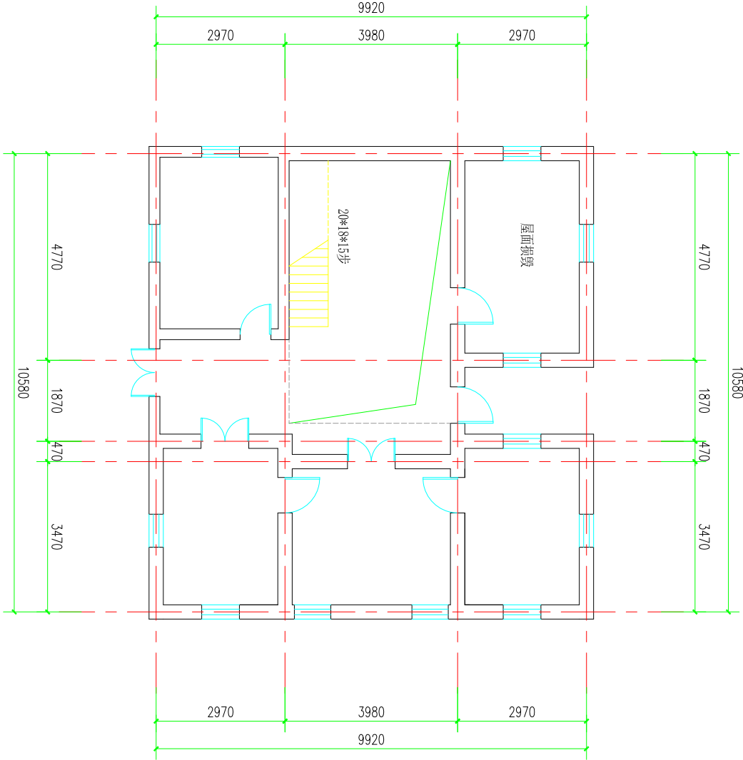
一层平面
