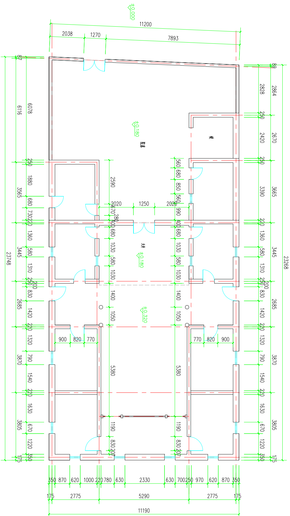
一层平面
