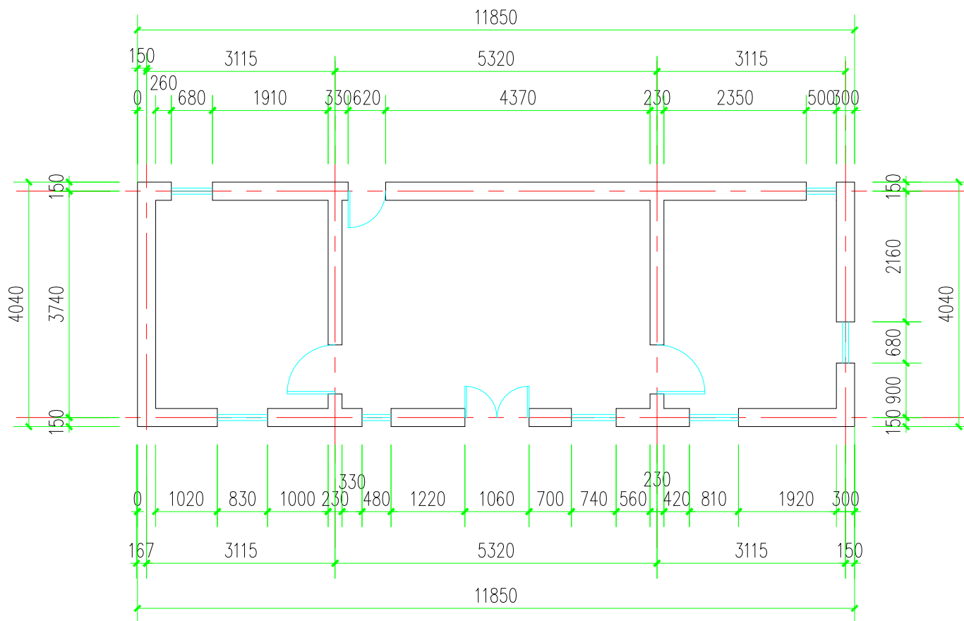
一层平面
