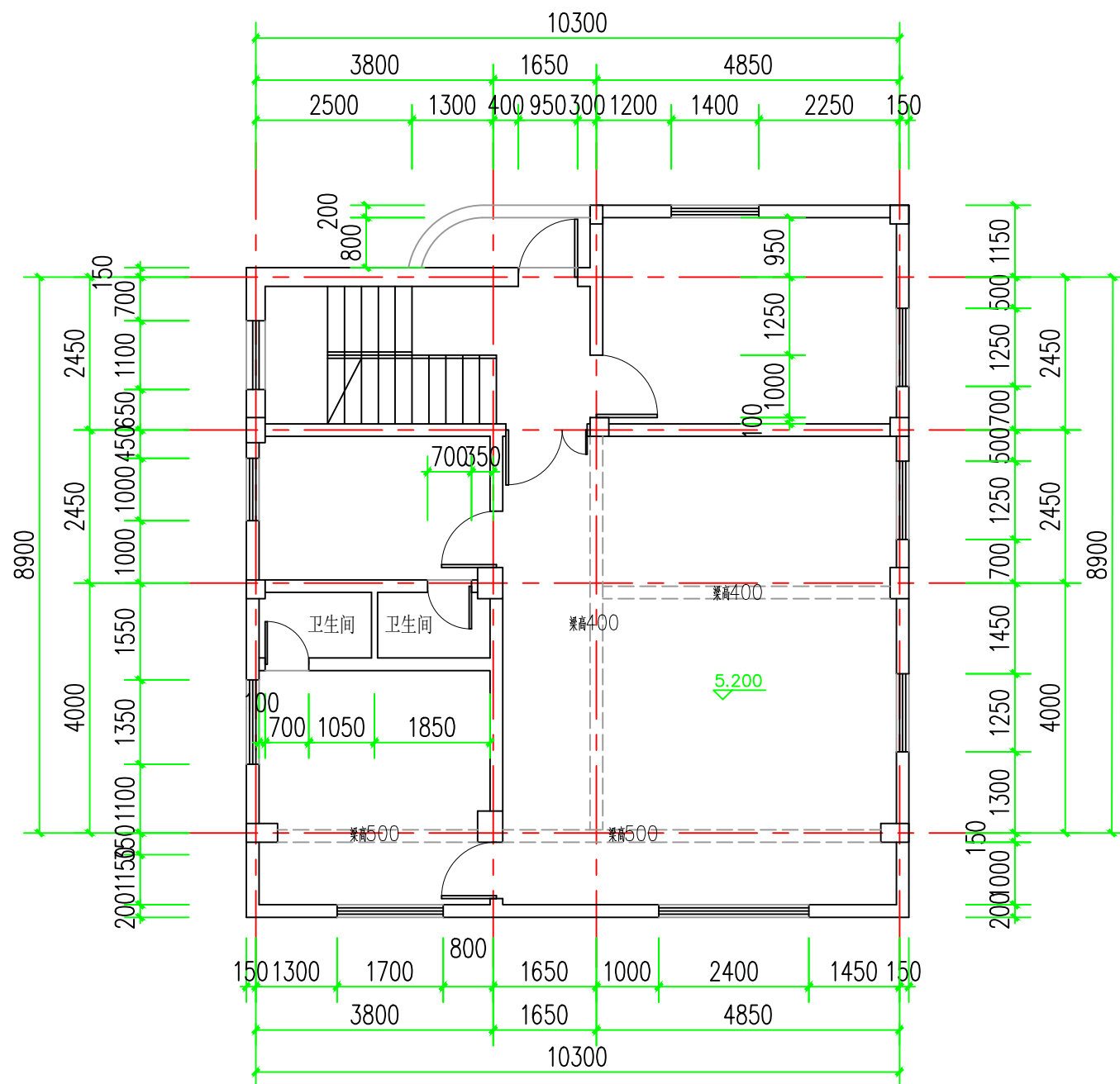
二层平面
