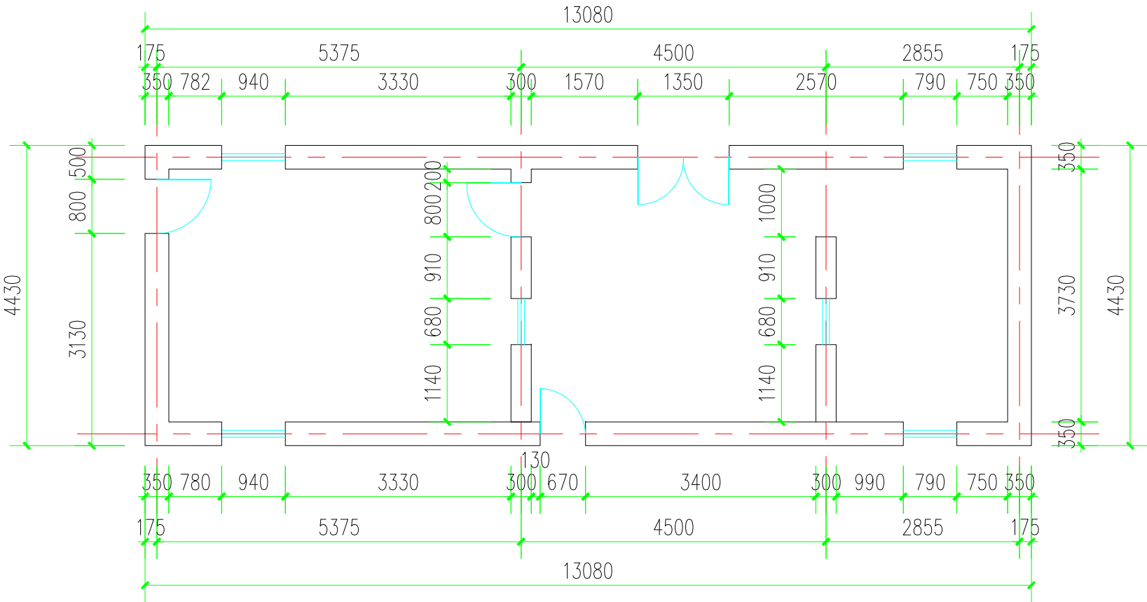
一层平面
