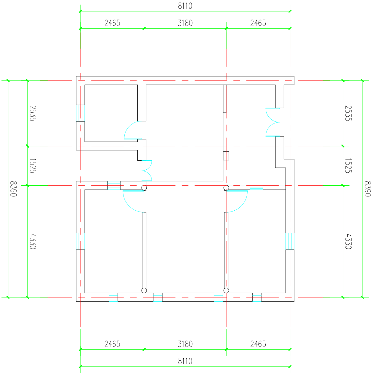
一层平面
