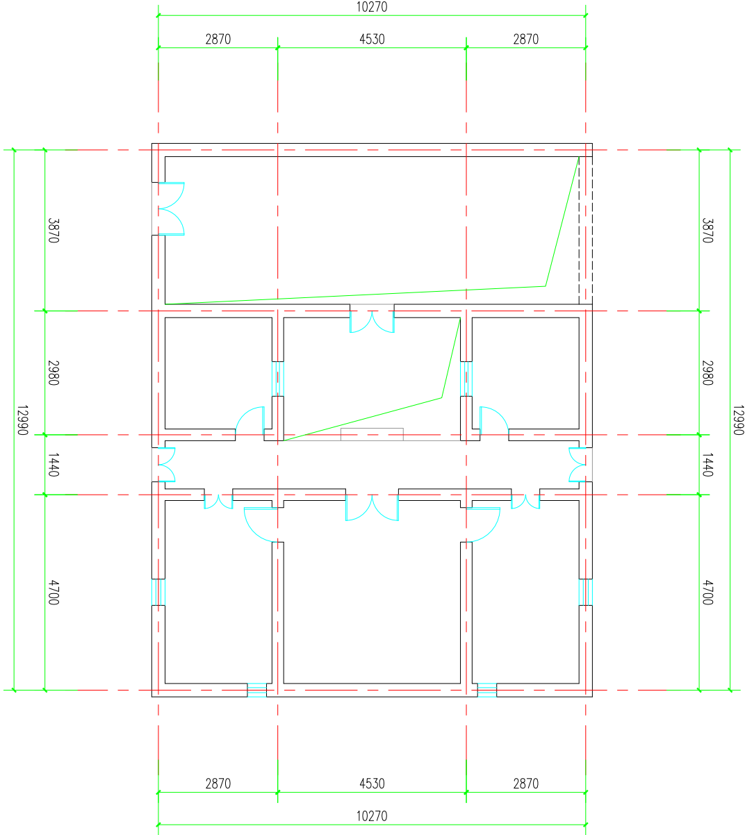
一层平面
