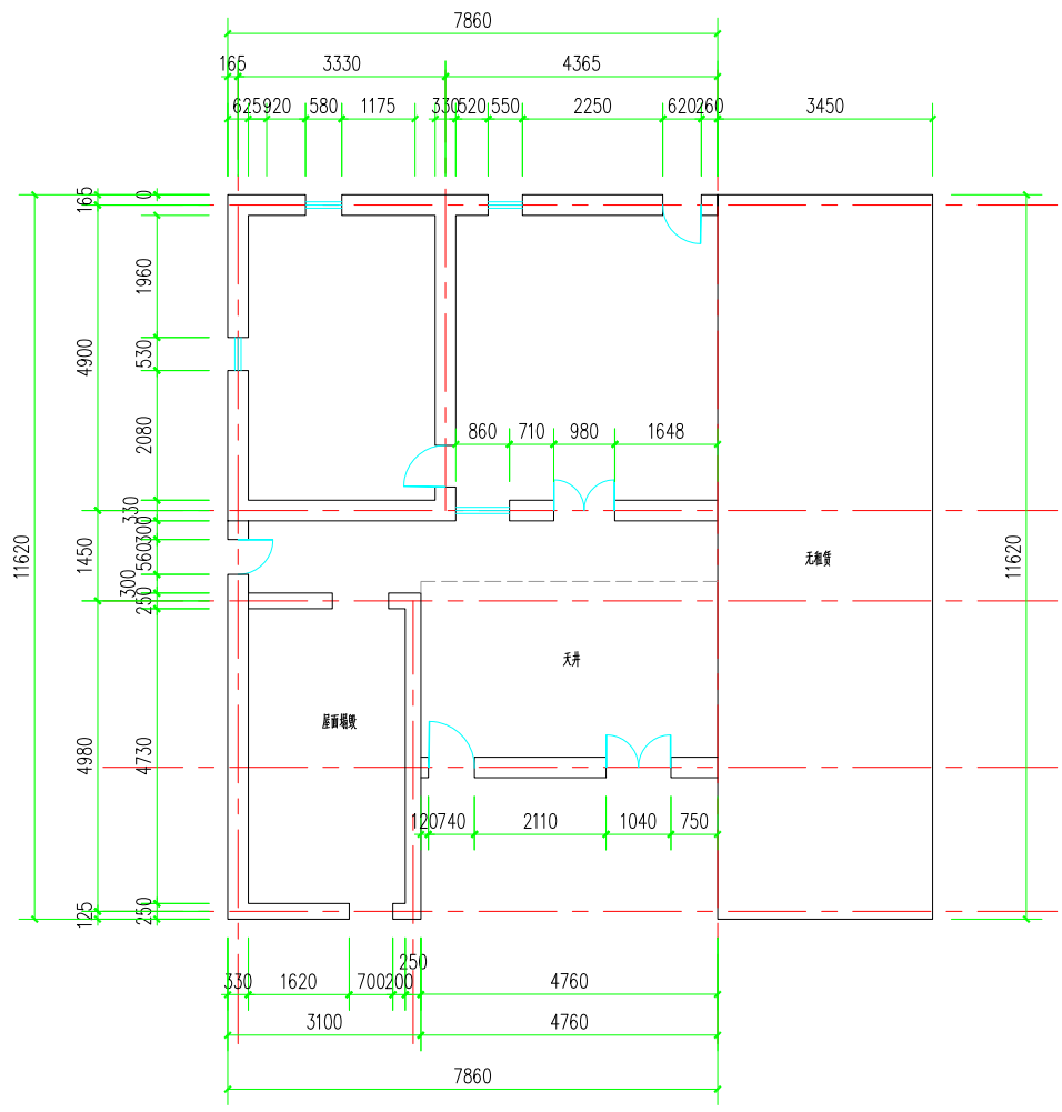
一层平面
