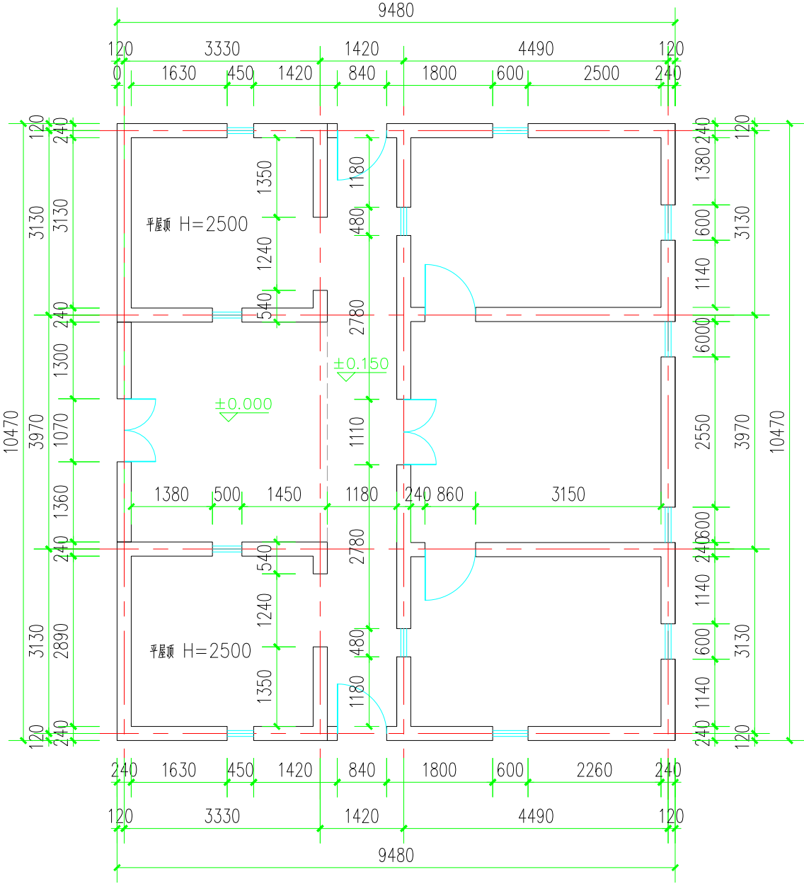
一层平面
