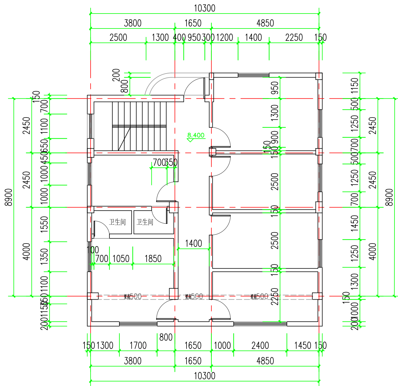
三层平面
