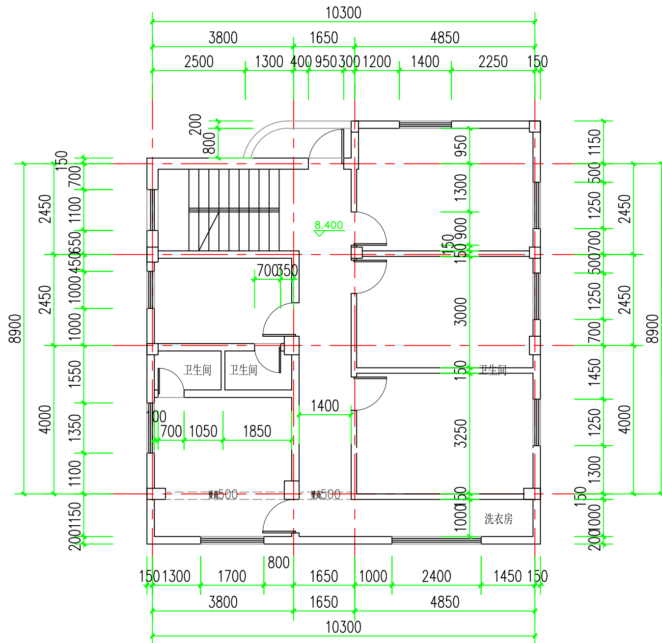
四层平面
