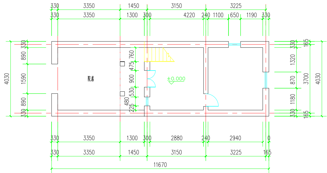
一层平面
