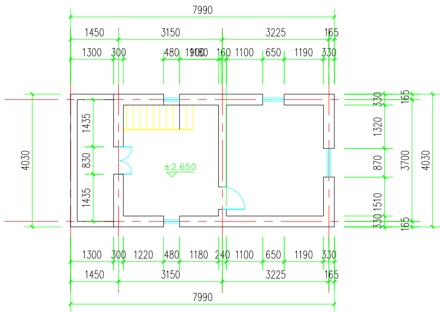
二层平面
