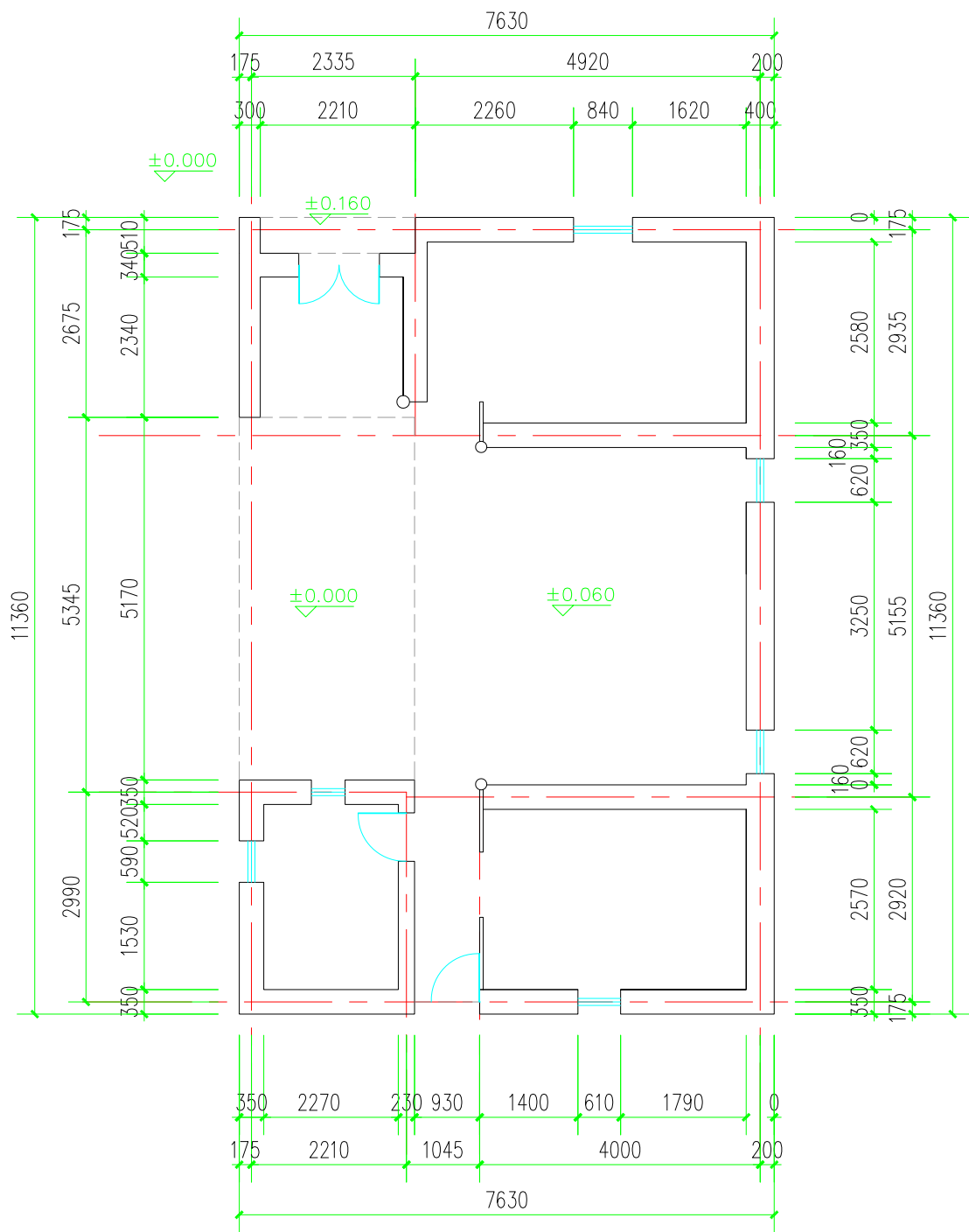
一层平面
