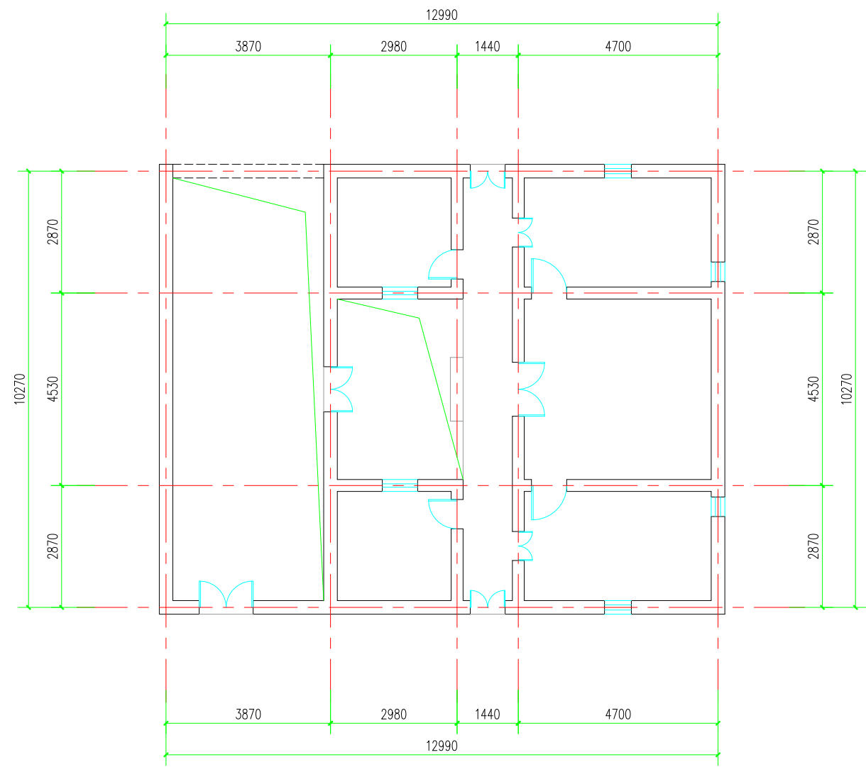
一层平面
