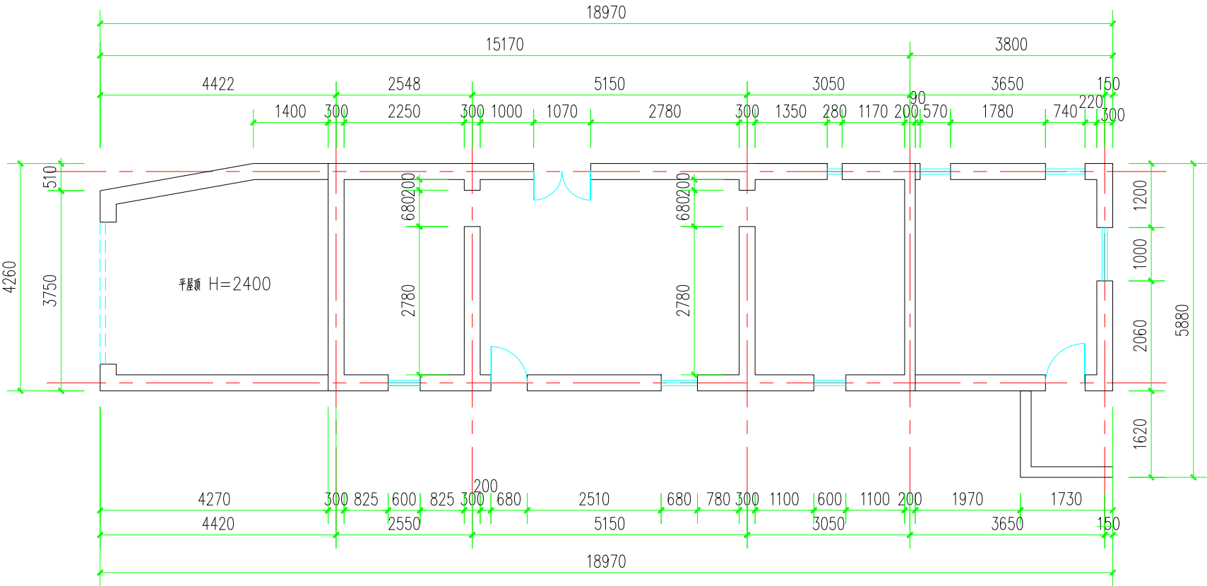
一层平面
