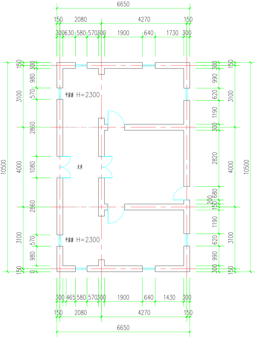
一层平面
