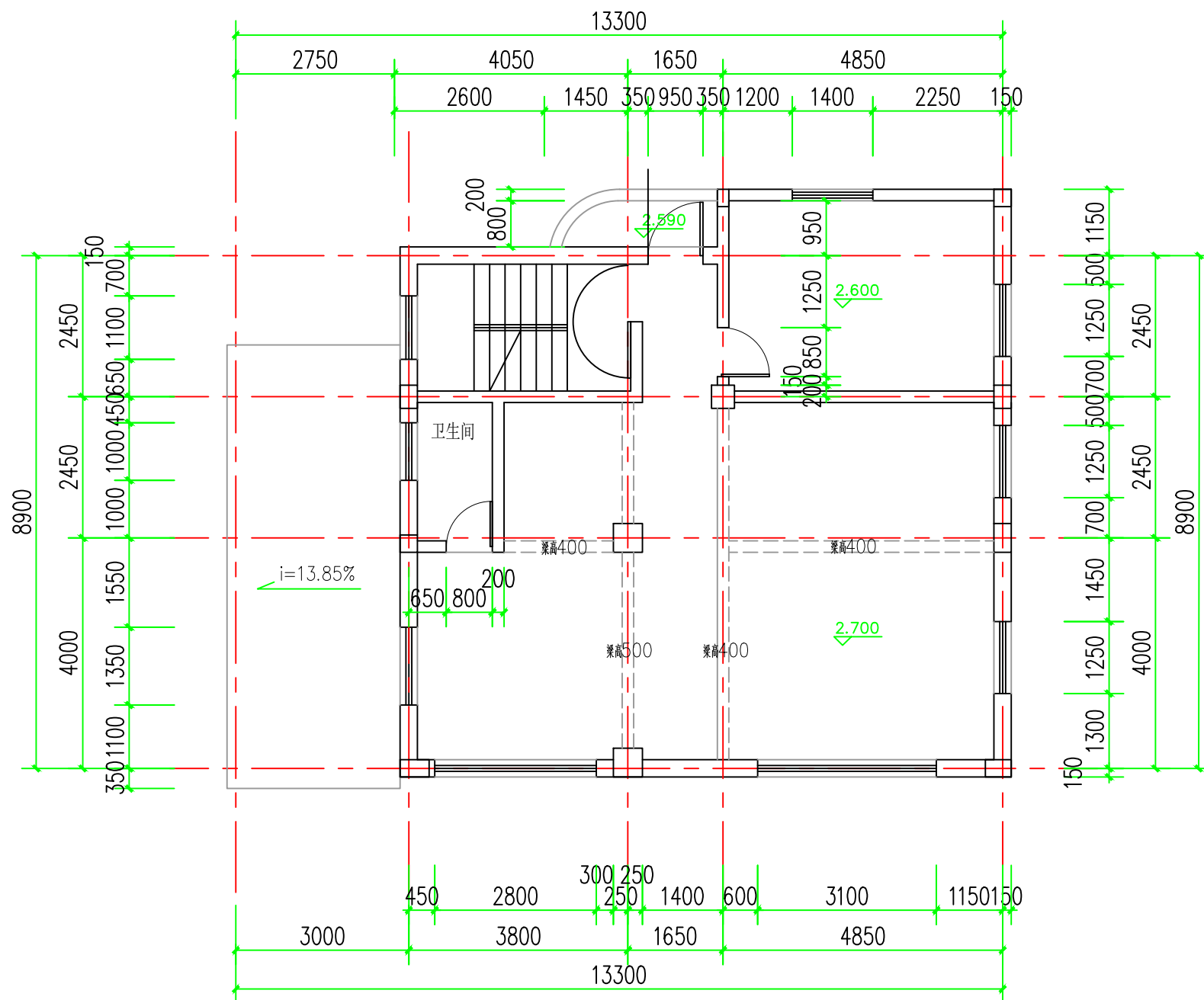
夹层平面
