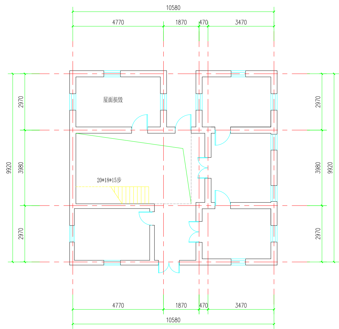
一层平面
