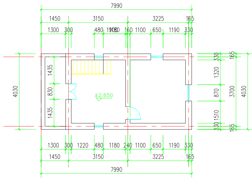
二层平面
