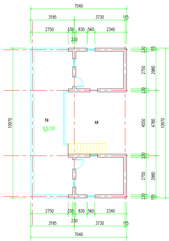
二层平面
