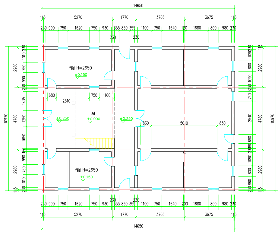
一层平面
