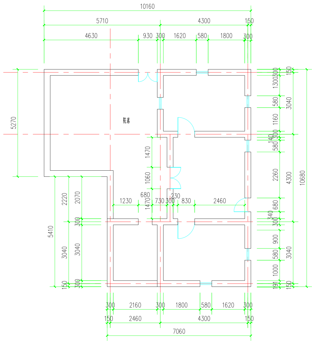
一层平面
