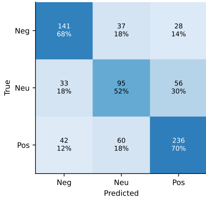
Valid
