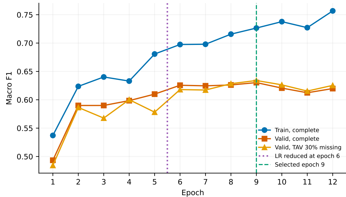
Macro F1
