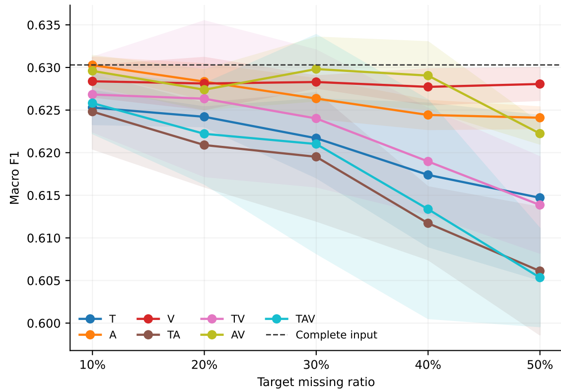
Macro F1
