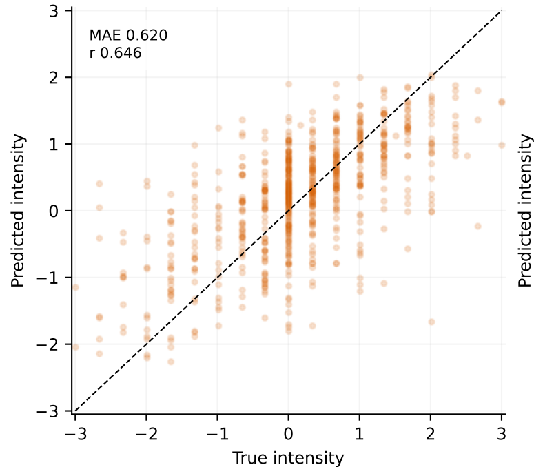
Valid · n=728
