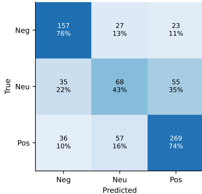
Test
