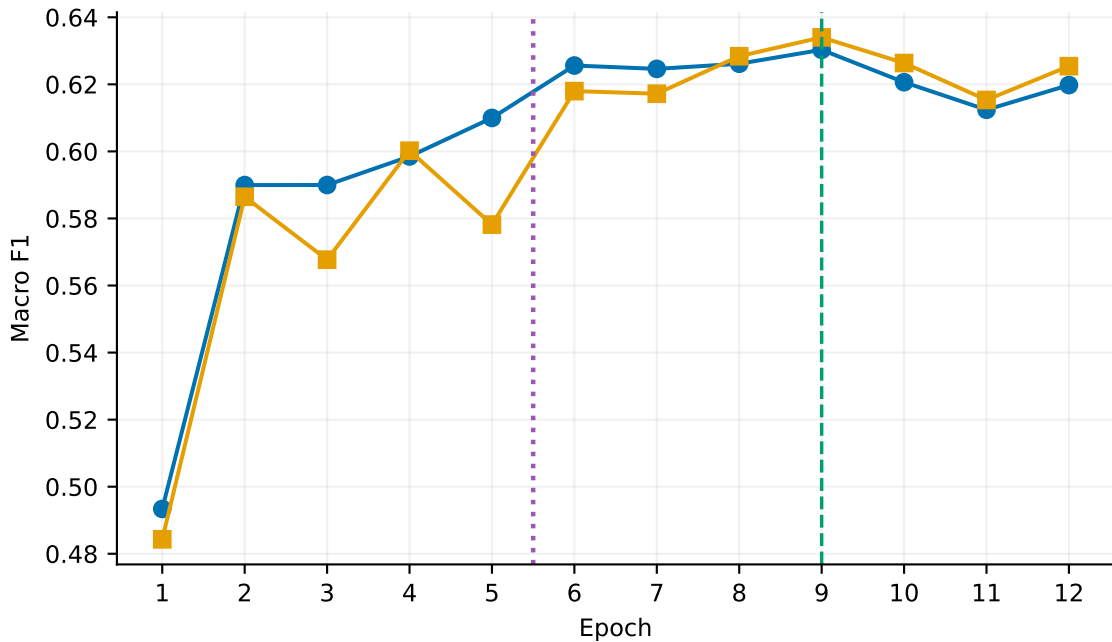
Macro F1
