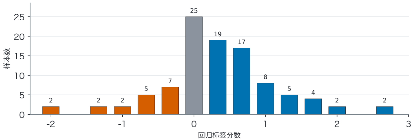
(c) 回归标签分布 (n=100)
