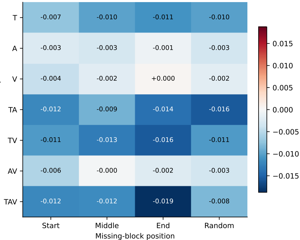
Change in Macro F1
