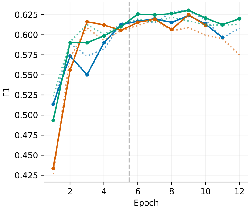
Validation Macro F1
