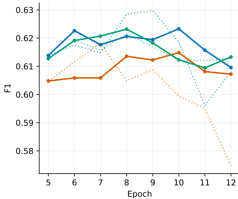
Validation Macro F1
