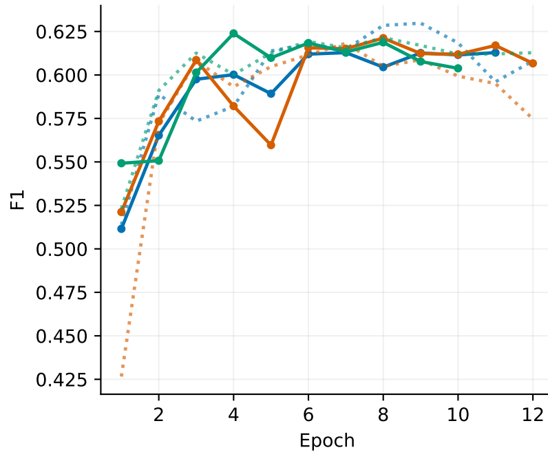
Validation Macro F1
