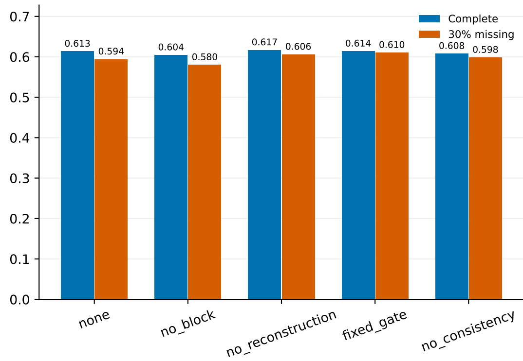
Macro F1
