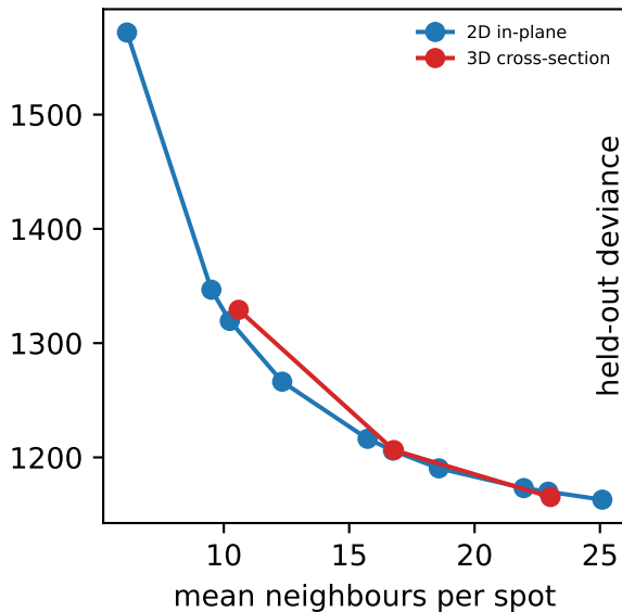
GSE214349 (label_um)
