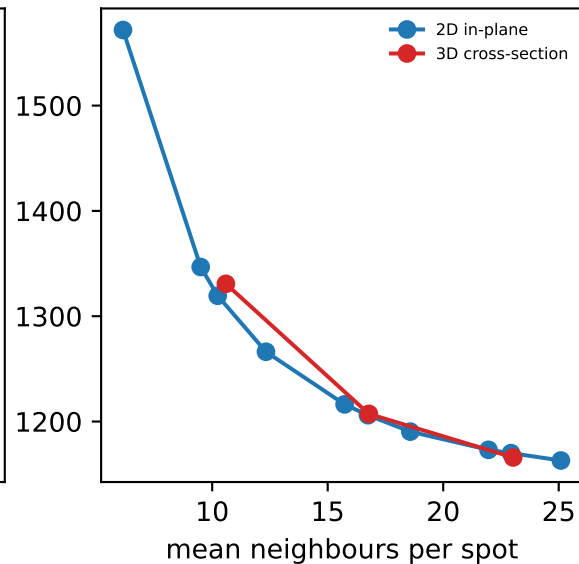
GSE214349 (order_x20um)
