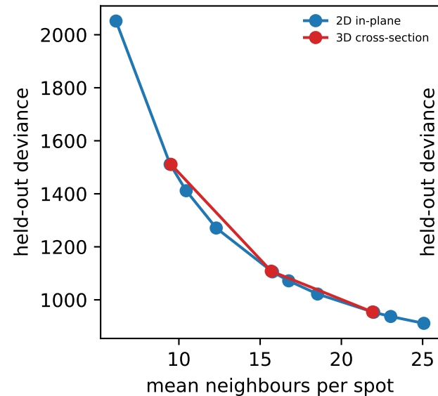
DLPFC_pairs (10um)
