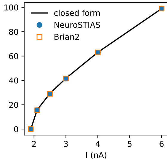
LIF f-I
