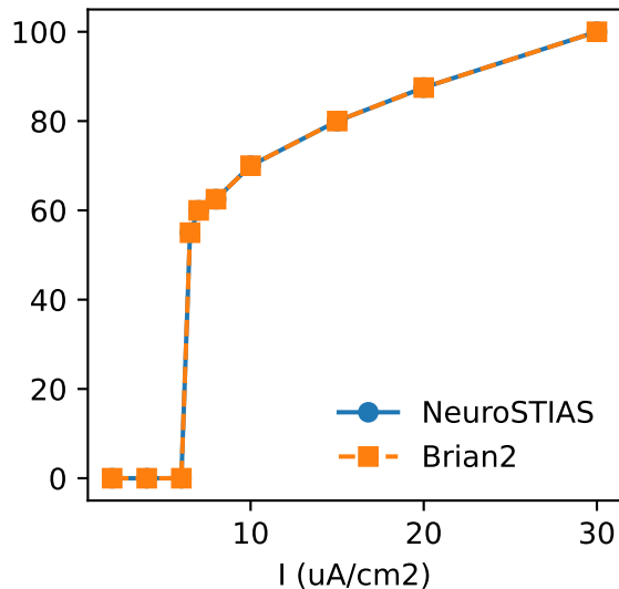
HH f-I
