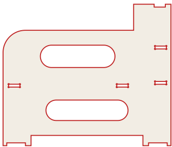
ARM-PANEL x2
