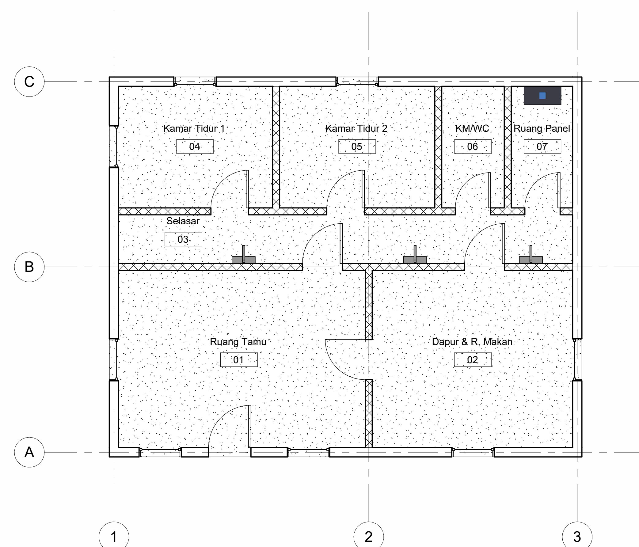
1 Denah Arsitektur - Lantai 1 1 : 50
