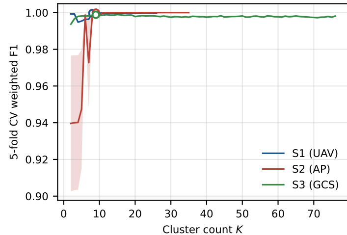
A: binary
