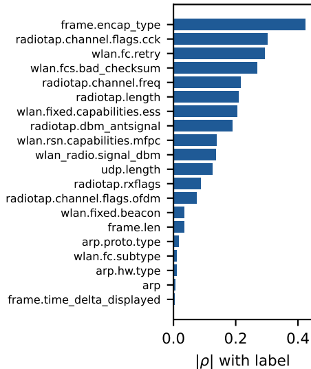
A: S1 (UAV), 20 features
