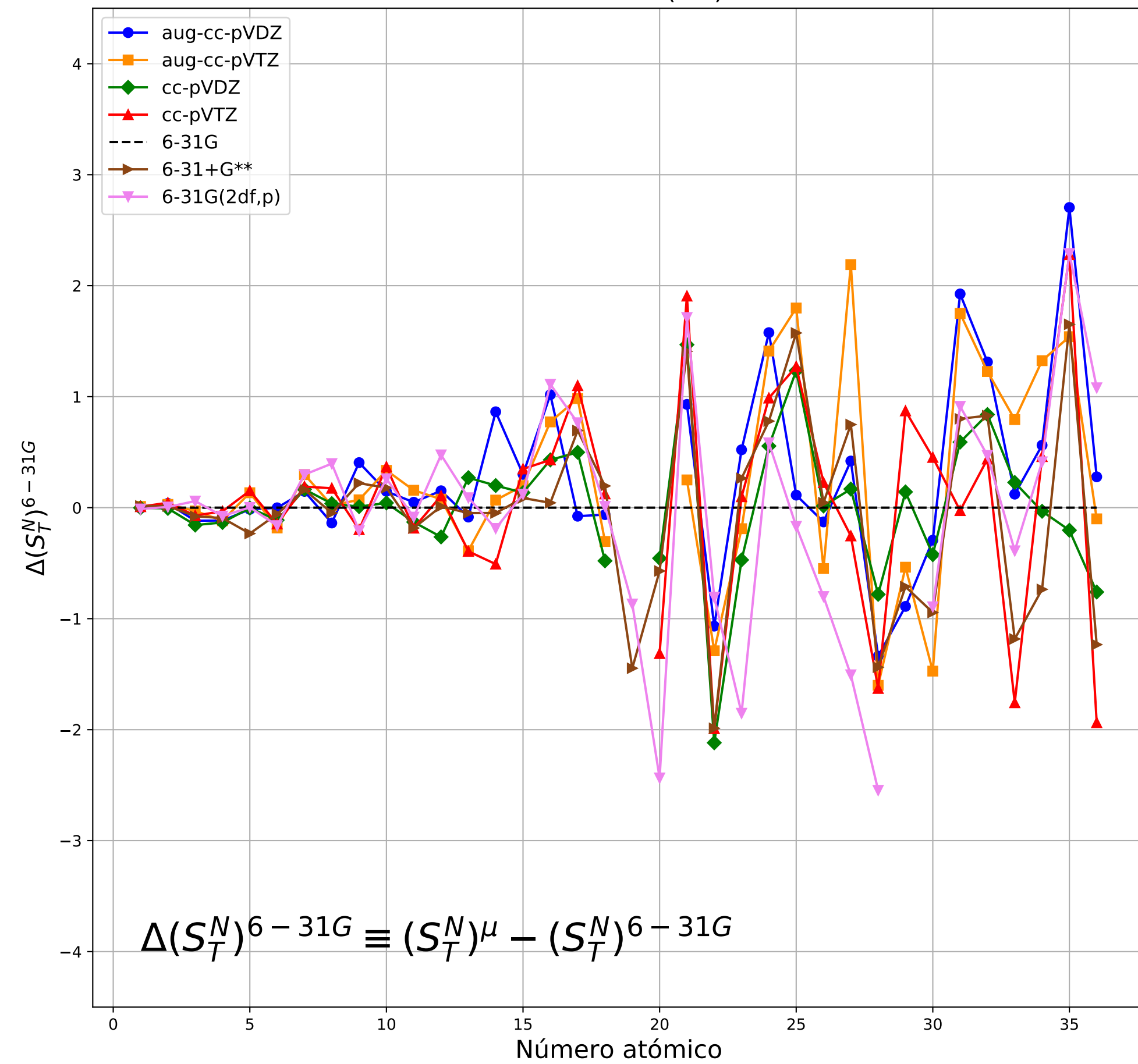
Método MP2(full)
