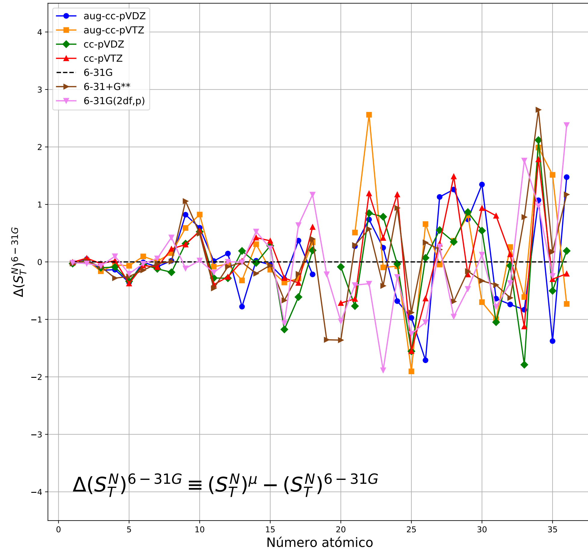
Método B3LYP
