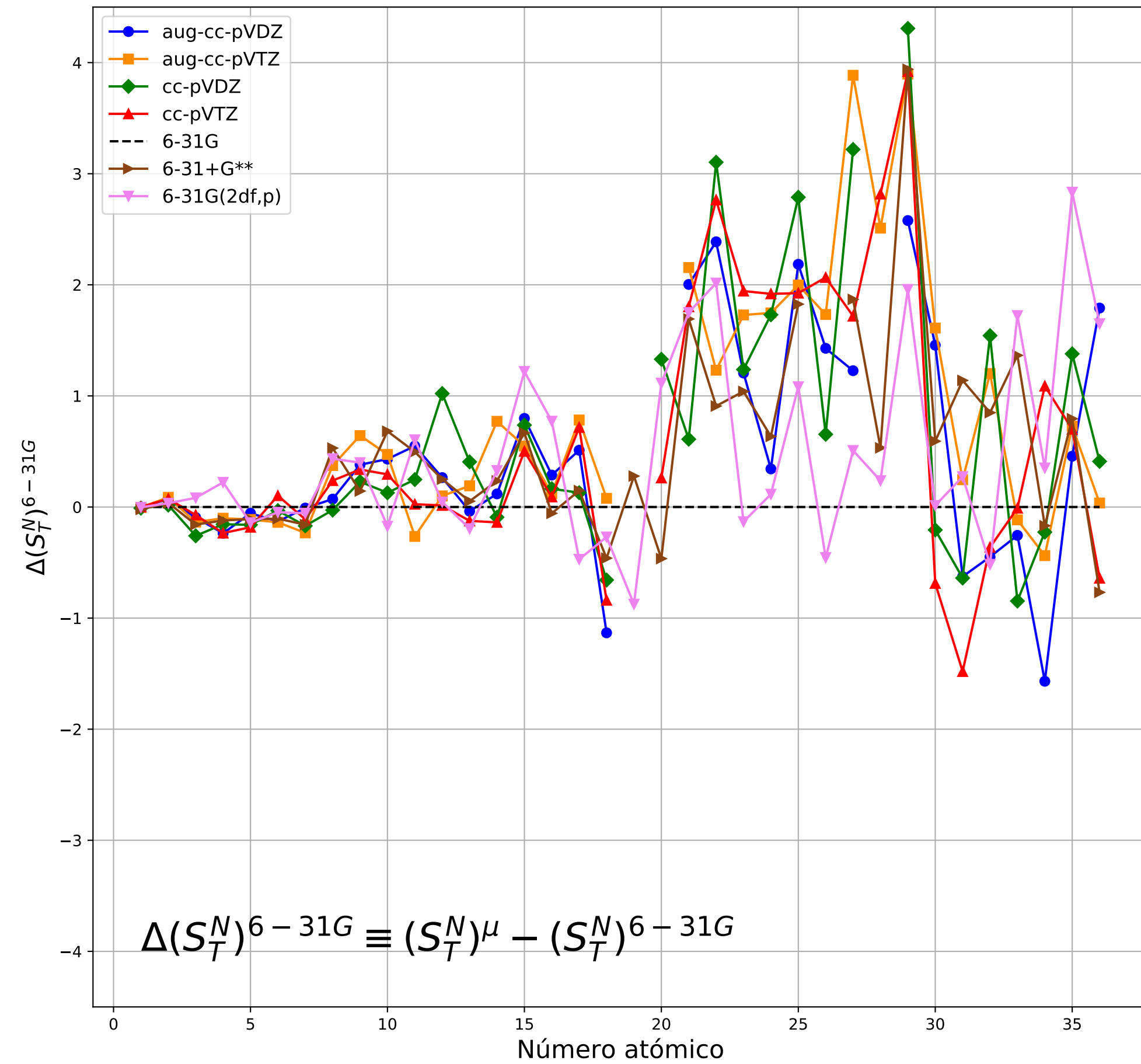
Método \omega B97X-D
