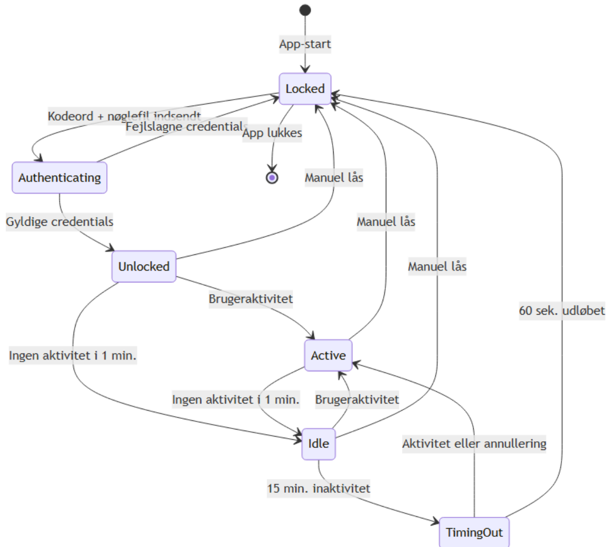
Figur 8.1: Session-livscyklus i Arx Runa. SessionKeys er mlockede i tilstandene Unlocked–TimingOut og zeroizes ved transition til Locked via ZeroizeOnDrop.
