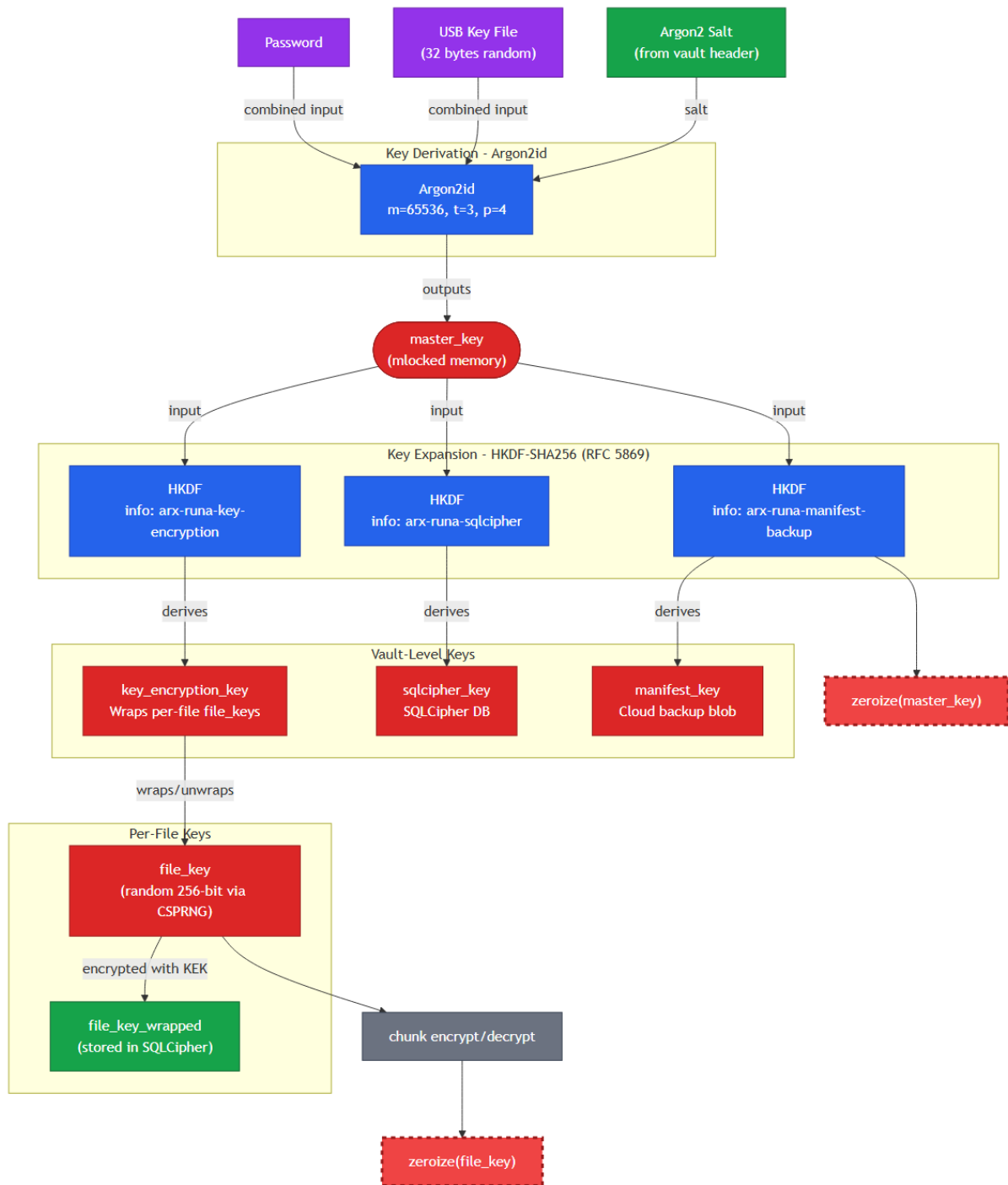
Figur 5.1: Nøgleafledningstre for Arx Runa. Adgangskode og USB-nøglefil kombineres som input til Argon2id ( m=65.536 , t=3 , p=4 ), der producerer master_key. HKDF-SHA256 ekspanderer master_key til tre vault-nøgler via domæneseparerede info-strengene. master_key zeroises lige efter HKDF-ekspansionen.
