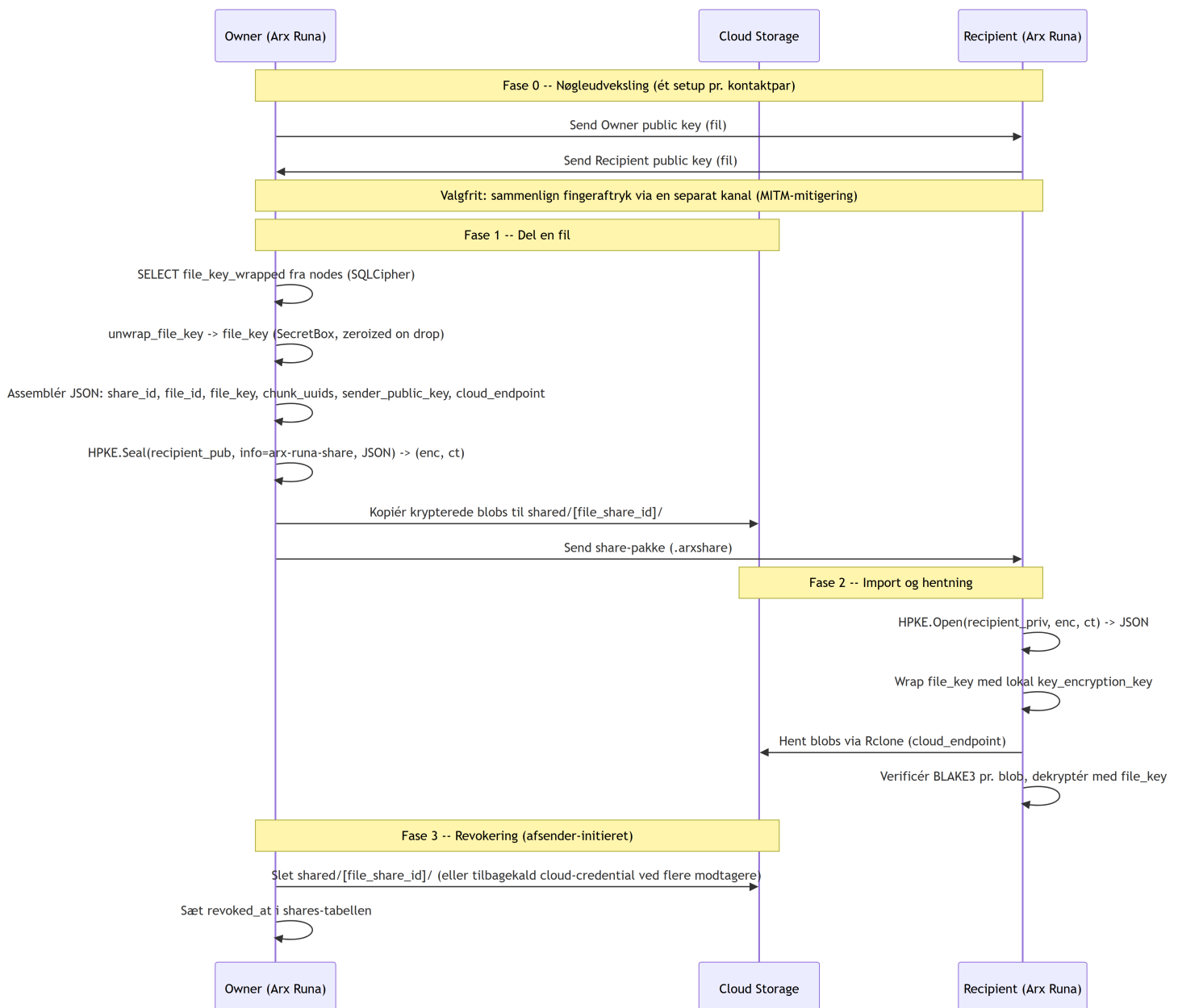
Figur 10.1: Det centrale delingsflow i Arx Runa. Fase 0 er et engangsetup pr. kontaktpar. Cloud-udbyderen modtager kun uigennemsigtige krypterede blobs og kan hverken læse indholdet eller identificere modtageren.
