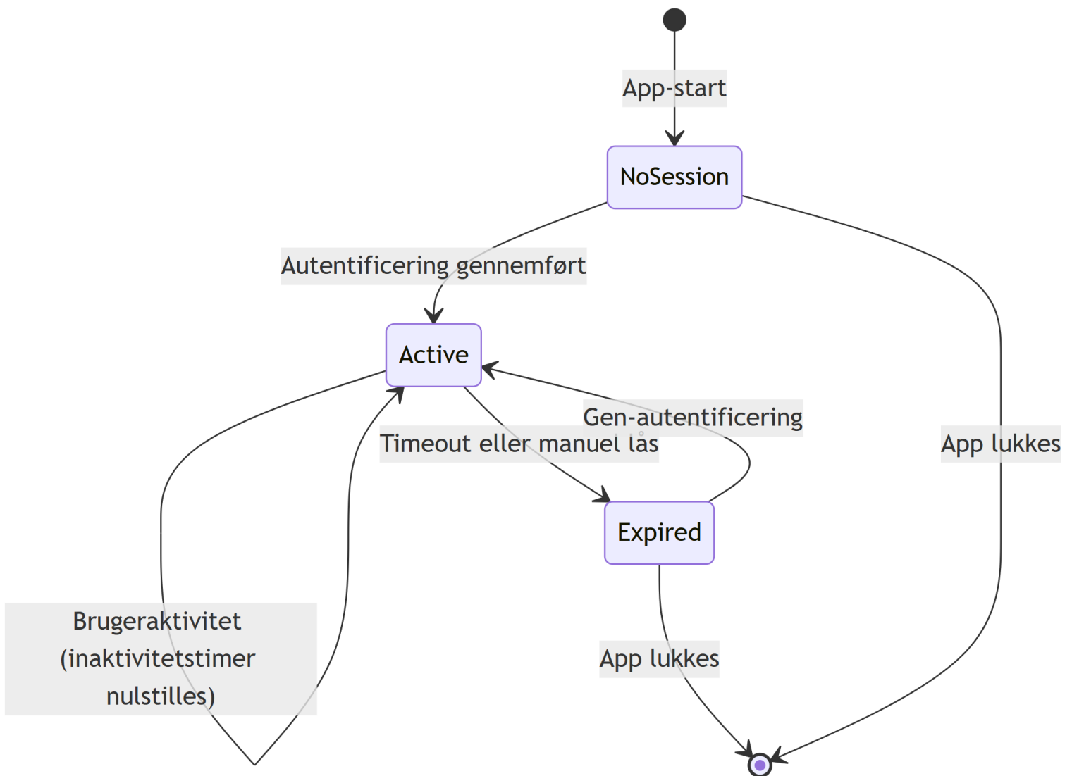
Figur 9.1: Session-livscyklus i Arx Runa. SessionKeys er mlocked i tilstanden Active og zeroizes ved overgangen til Expired . En TimeoutWarning { seconds_remaining } -hændelse emitteret via intern broadcast-kanal kort før automatisk lås.
