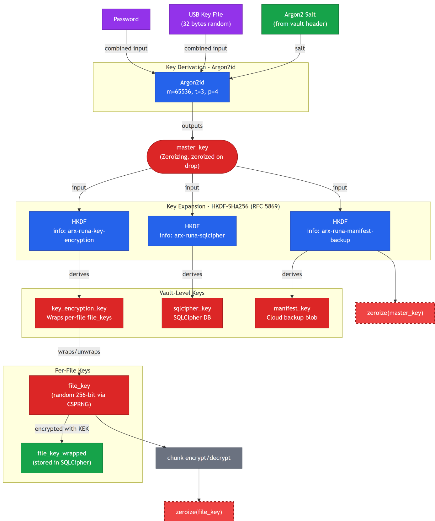
Figur 6.1: Nøgleafledningstre for Arx Runa. Adgangskode og USB-nøglefil kombineres som input til Argon2id ( m=65.536 , t=3 , p=4 ), der producerer master_key. HKDF-SHA256 ekspanderer master_key til tre vault-nøgler via domæneseparerede info-strengene. master_key zeroises lige efter HKDF-ekspansionen.
