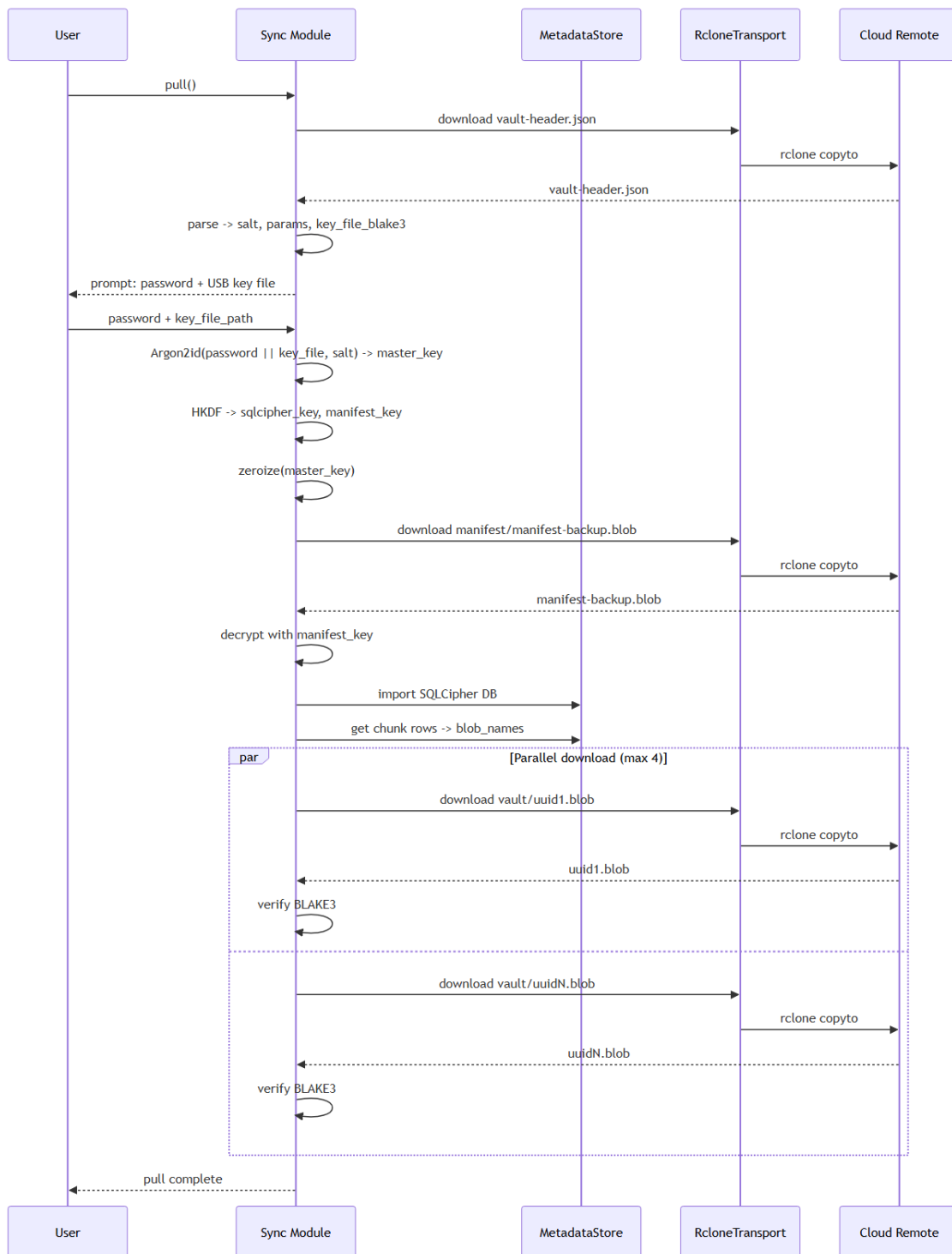
Figur 8.4: Pull-flow (ny-enhed recovery). Vault-header hentes og bruges til nøgleafledning; manifest-backup dekrypteres og importeres; alle blobs downloades og BLAKE3-verificeres.
