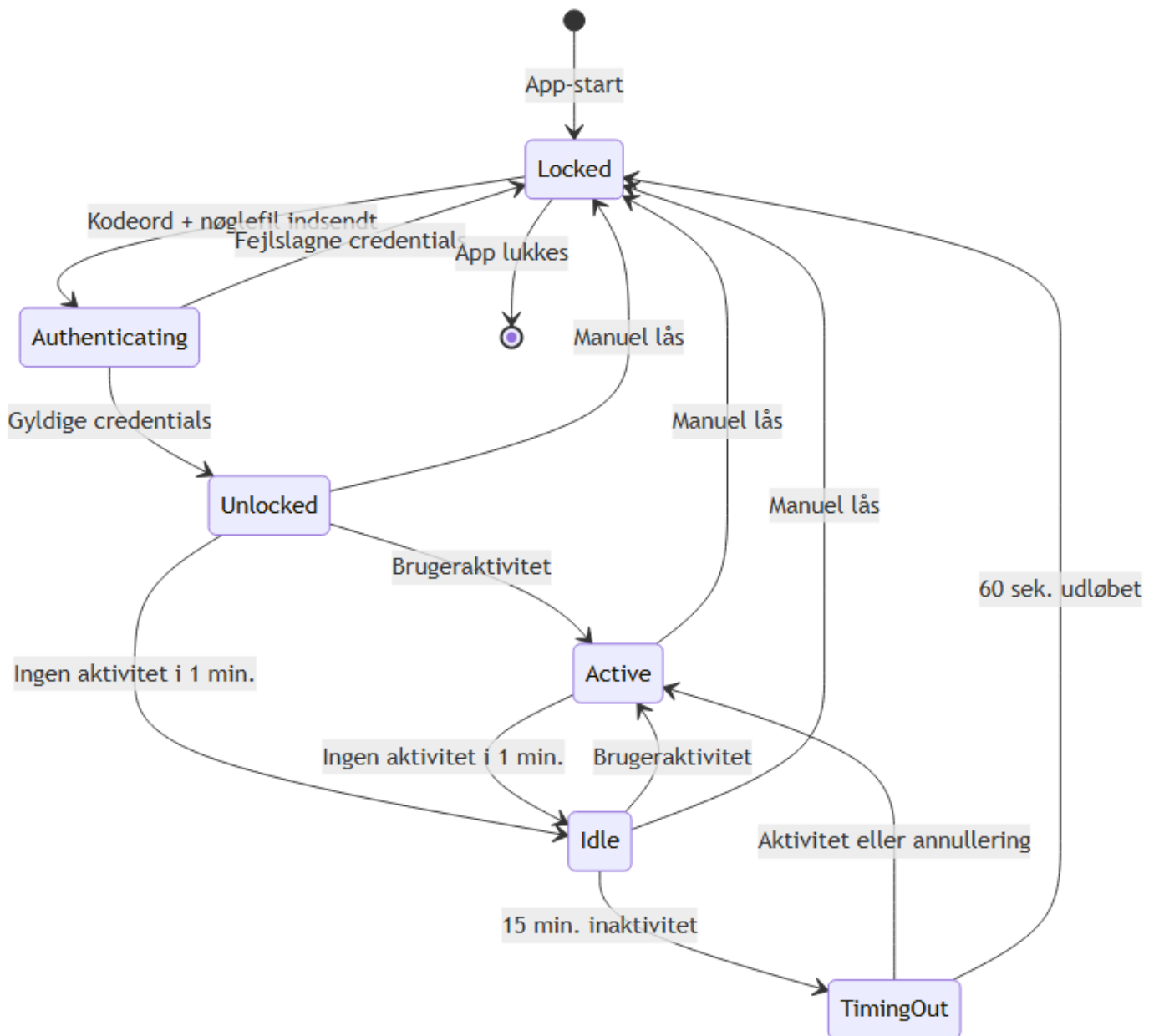
Figur 9.1: Session-livscyklus i Arx Runa. SessionKeys er mlocked i tilstandene Unlocked–TimingOut og zeroizes ved transition til Locked via ZeroizeOnDrop.
