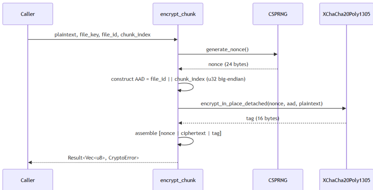
Figur 6.2: Krypteringsflow for ét chunk med CSPRNG-nonce, AAD-binding og wire-format [nonce | ciphertext | tag].
