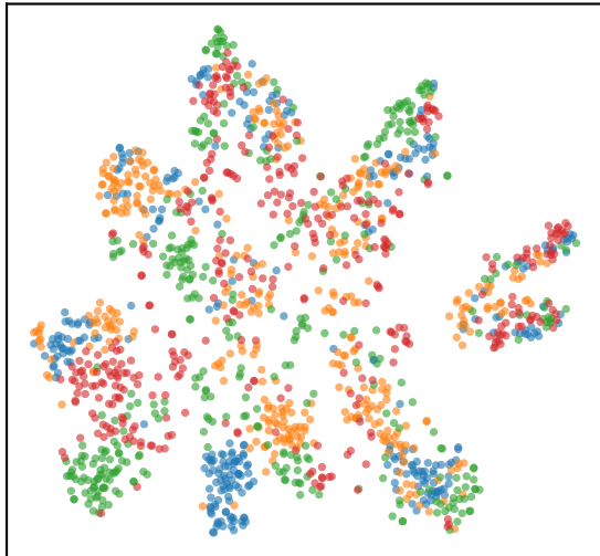
dan
