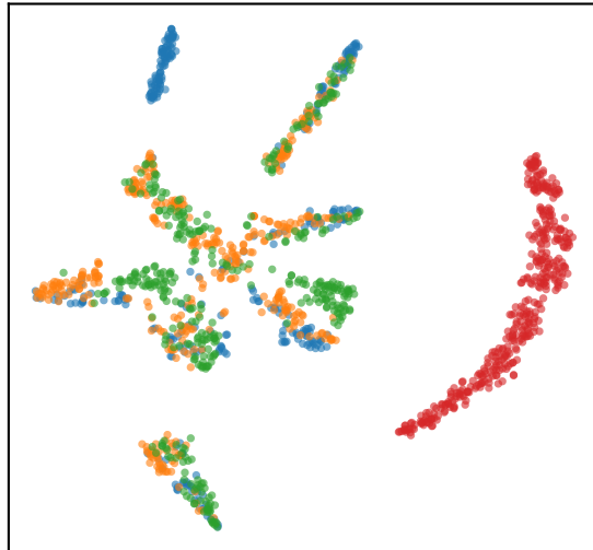
dann
