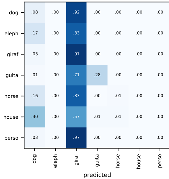
dann (acc 0.248)
