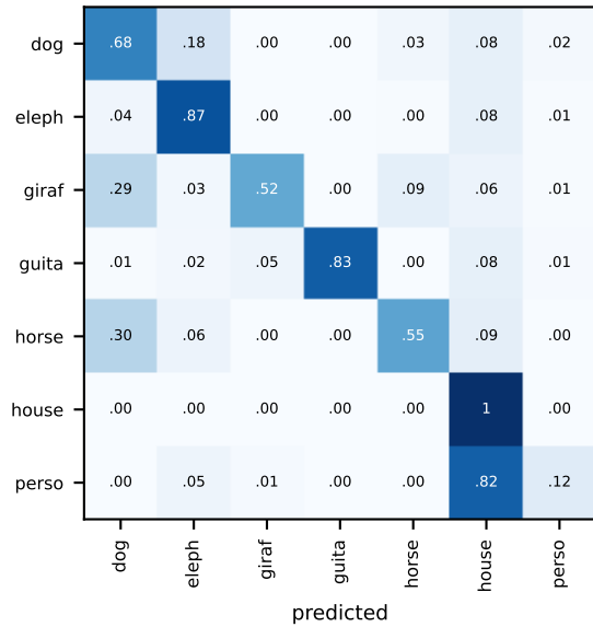
cdan (acc 0.665)
