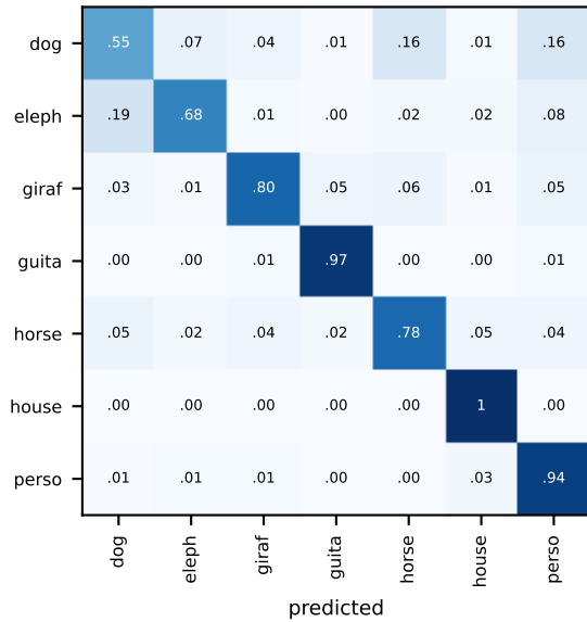
dan (acc 0.758)
