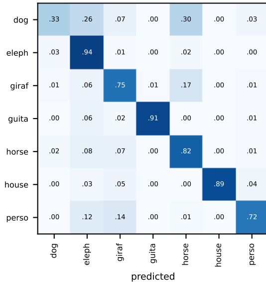
sam (acc 0.742)
