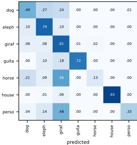
erm (acc 0.572)
