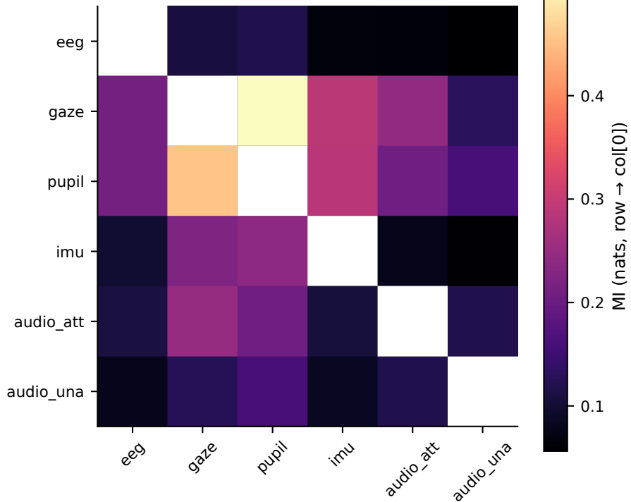
Mutual information (Subject 1 · Eval-6)
