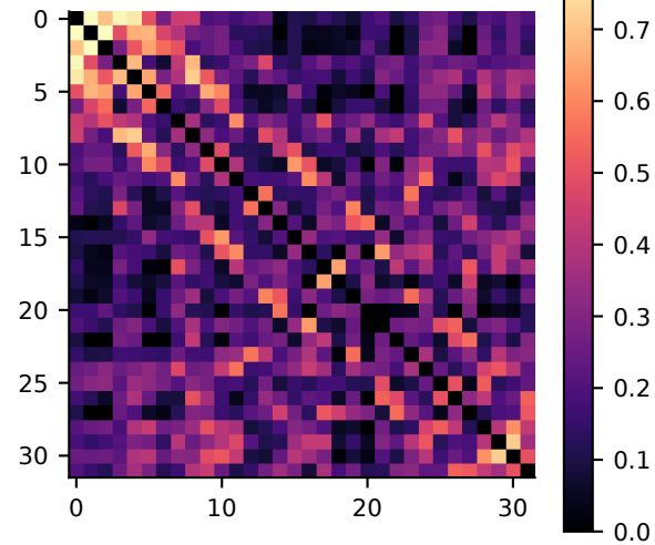
AEC · 8-13 Hz · S1E6
