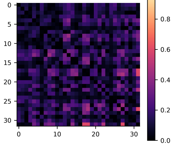
wPLI · 8-13 Hz · S1E6
