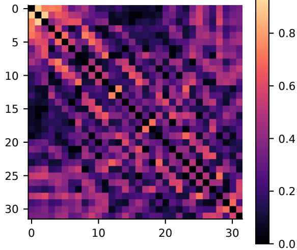
PLV · 8-13 Hz · S1E6
