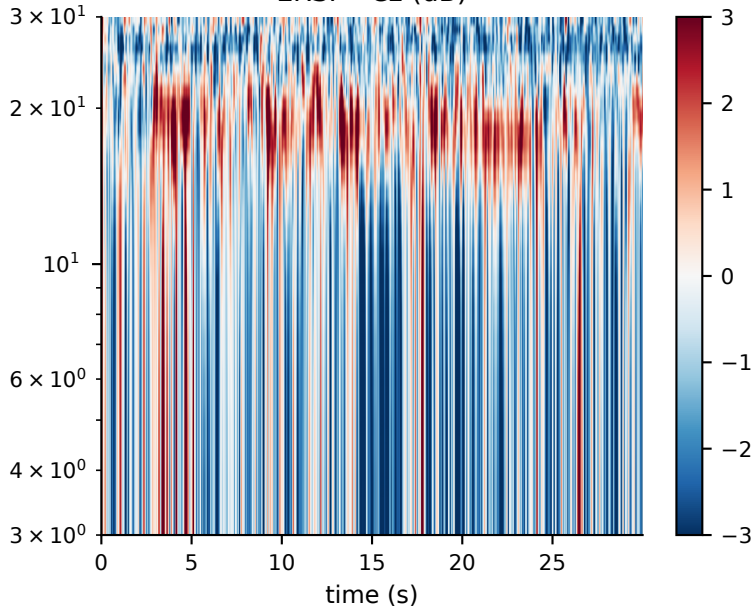
ERSP · Cz (dB)
