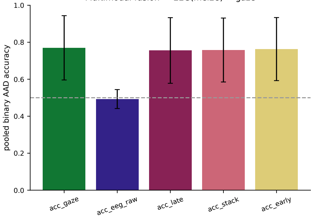
Multimodal fusion — EEG(mel28) × gaze
