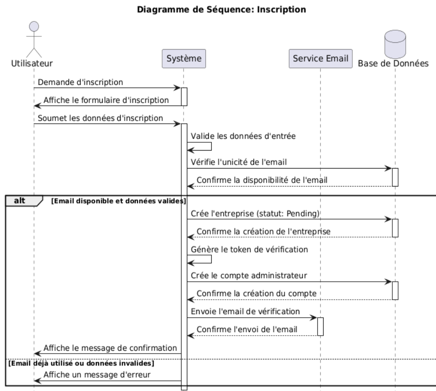
FIGURE 4.6 – Diagramme de séquence pour le scénario d'inscription
