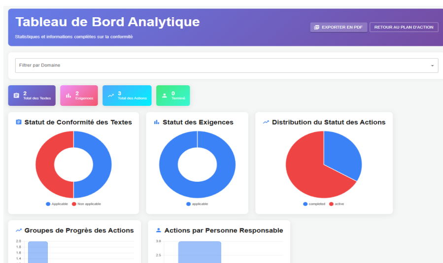
FIGURE 5.58 – Interface des statistiques de conformité
