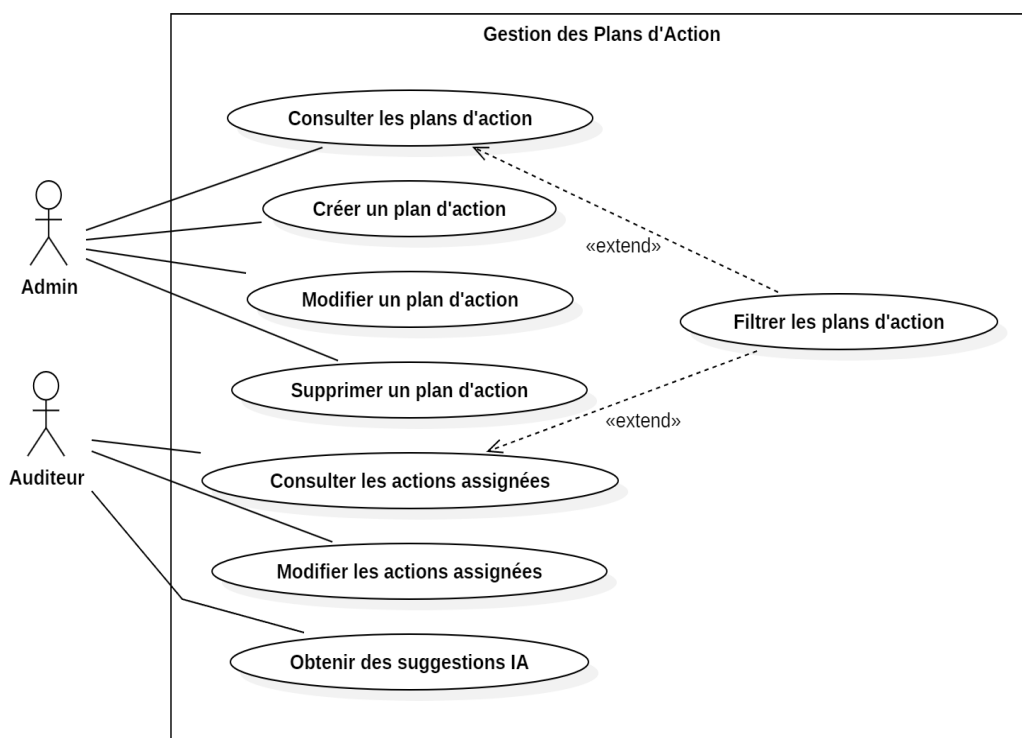
FIGURE 5.5 – Diagramme de cas d'utilisation - Gestion des plans d'action
