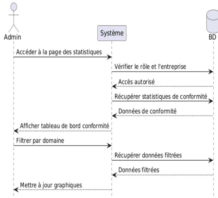
FIGURE 5.50 – Diagramme de séquence pour le scénario de consultation des statistiques de conformité
