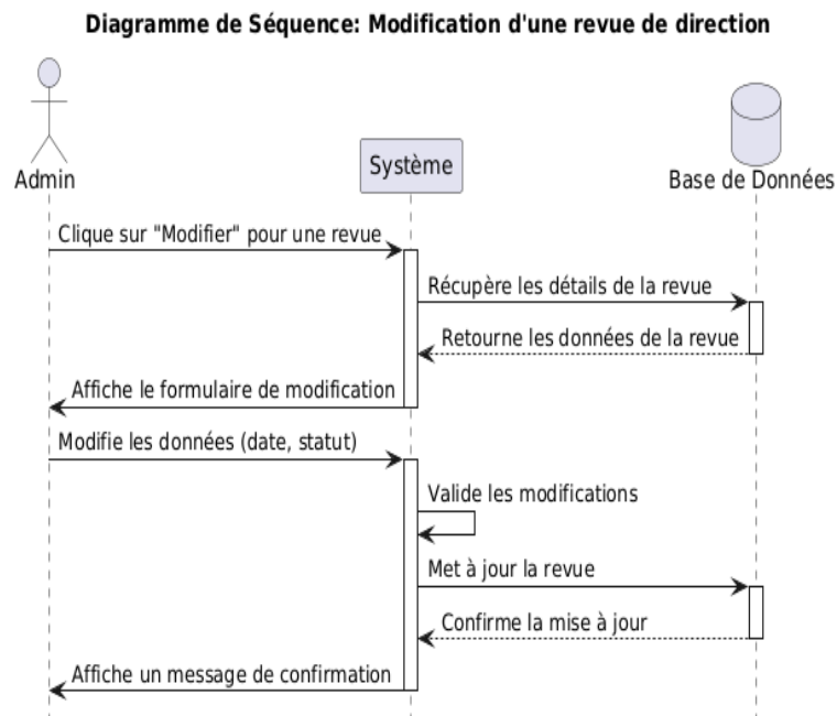
FIGURE 5.38 – Diagramme de séquence pour le scénario de modification d'une revue de direction
