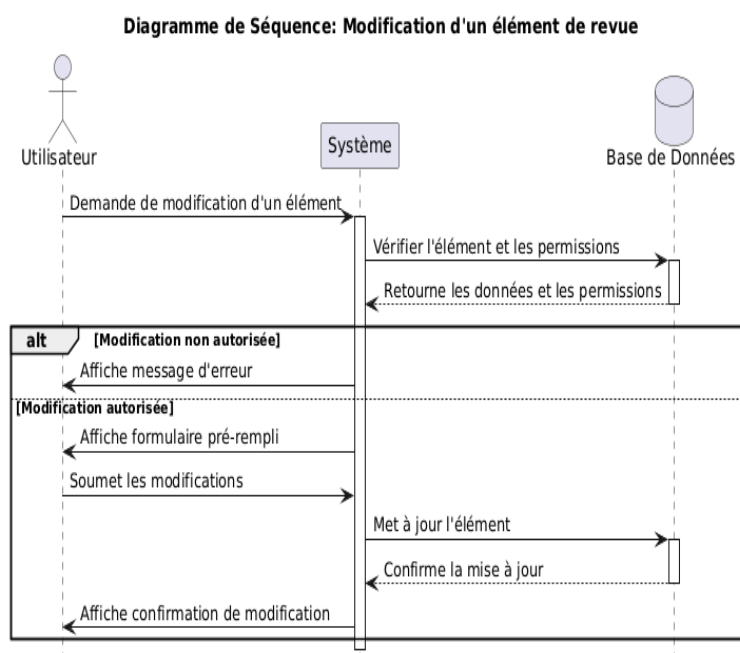
FIGURE 5.43 – Diagramme de séquence pour le scénario de modification d'un élément de revue
