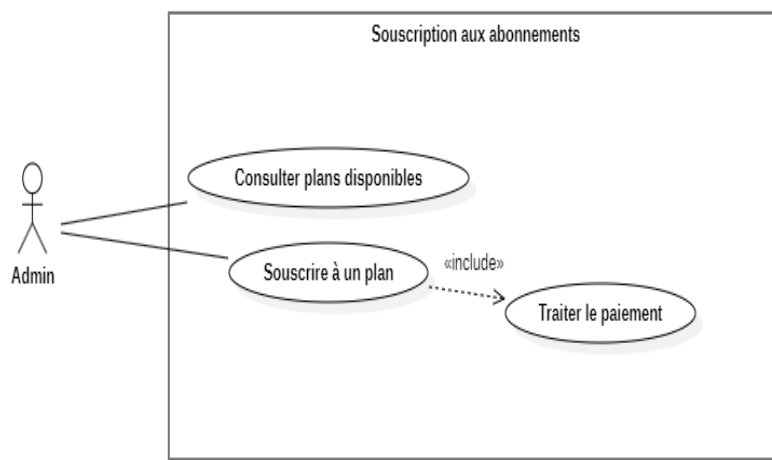
FIGURE 5.2 – Diagramme de cas d'utilisation - Souscription aux abonnements
