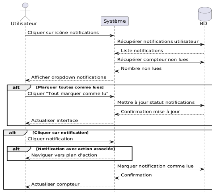
FIGURE 5.46 – Diagramme de séquence pour le scénario de consultation des notifications
