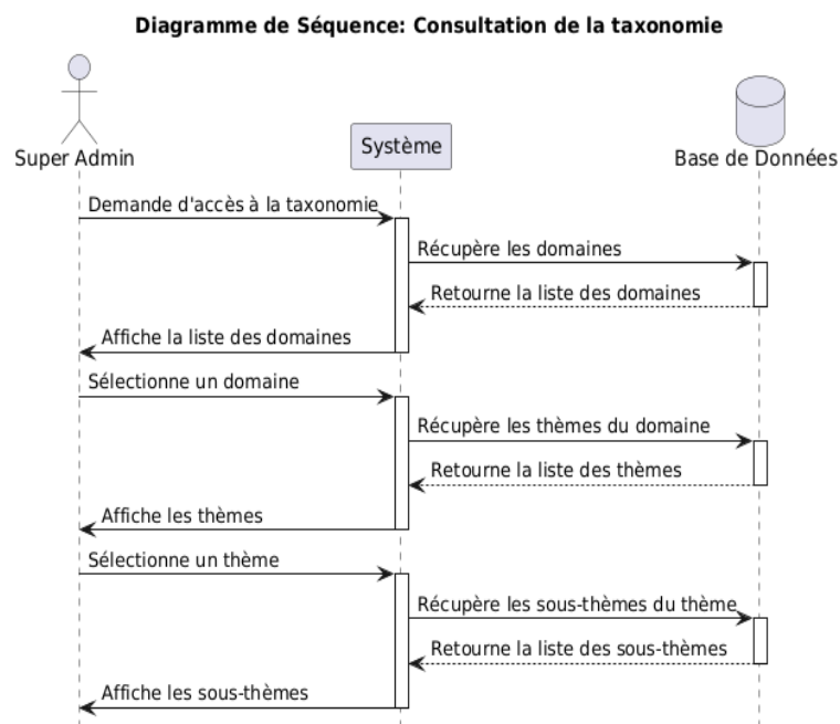
FIGURE 4.26 – Diagramme de séquence pour le scénario de consultation de la taxonomie
