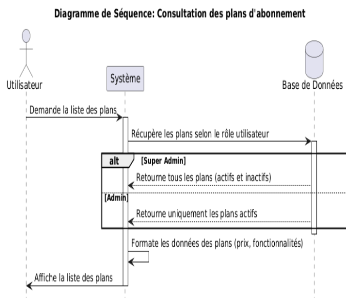
FIGURE 5.7 – Diagramme de séquence pour le scénario de consultation des plans d'abonnement
