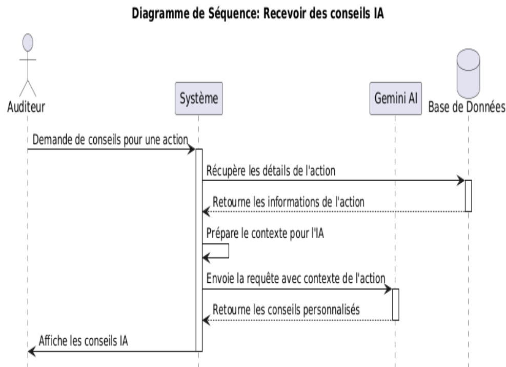
FIGURE 5.20 – Diagramme de séquence pour le scénario de génération de conseils IA
