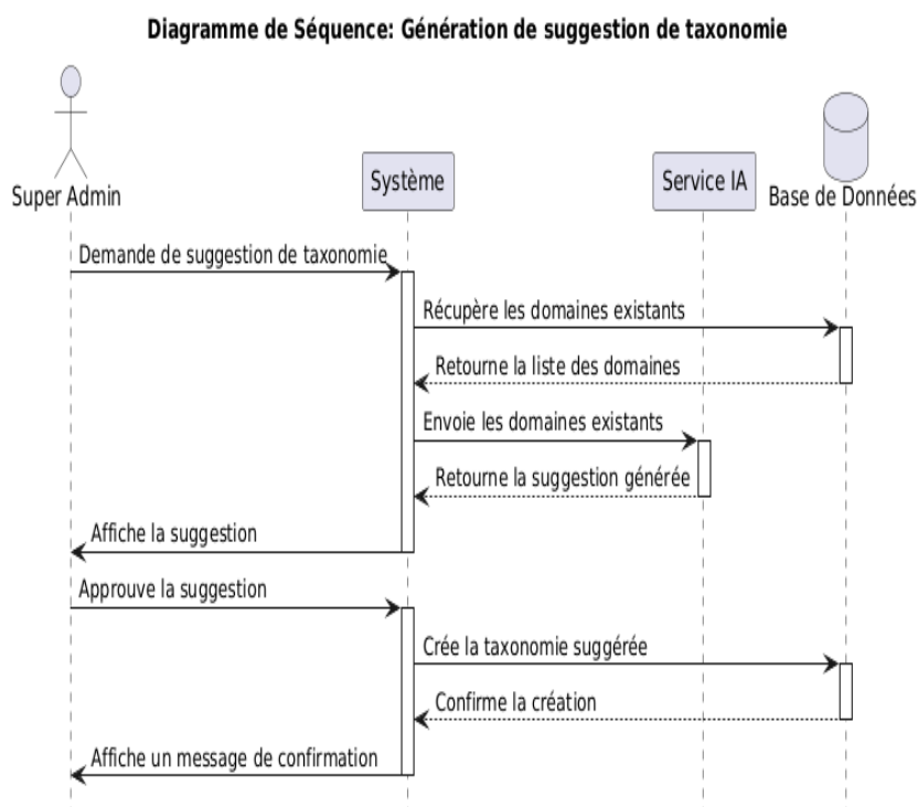
FIGURE 4.29 – Diagramme de séquence pour le scénario de génération de suggestion de taxonomie
