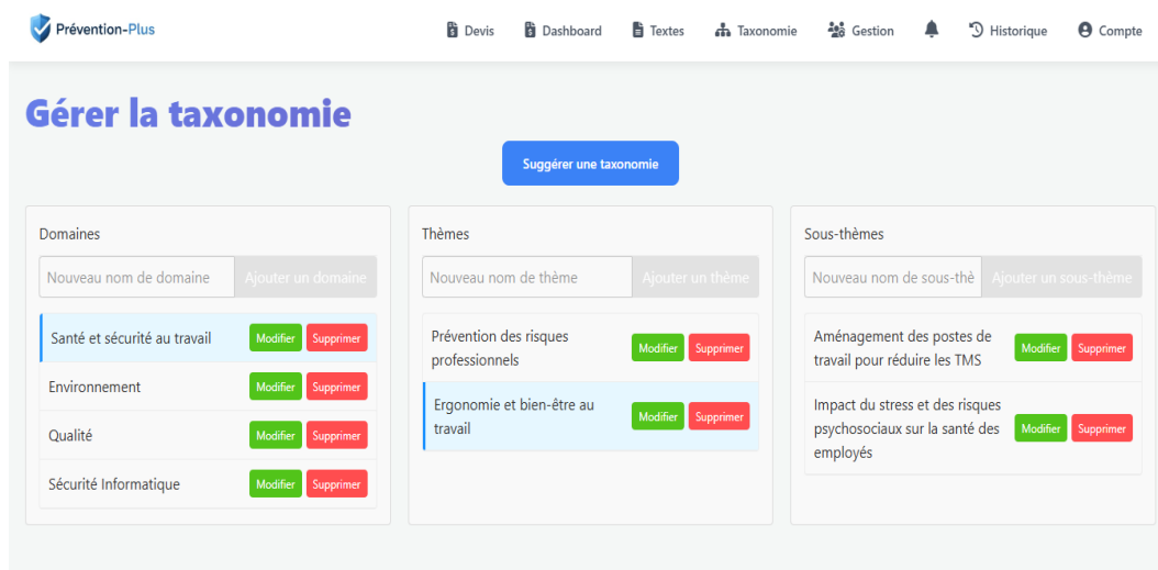
FIGURE 4.36 – Interface de gestion de la taxonomie
