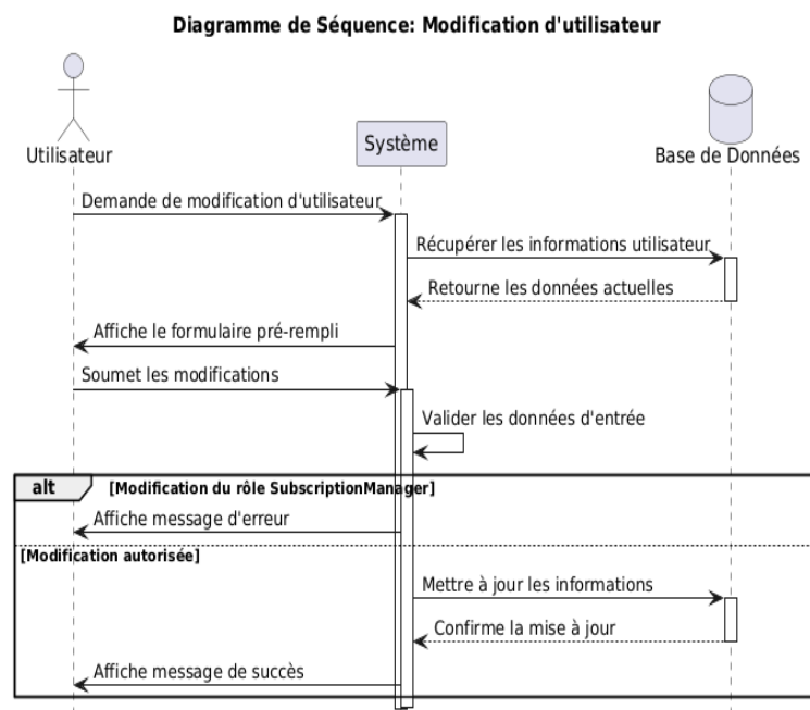
FIGURE 4.19 – Diagramme de séquence pour le scénario de modification d'utilisateur
