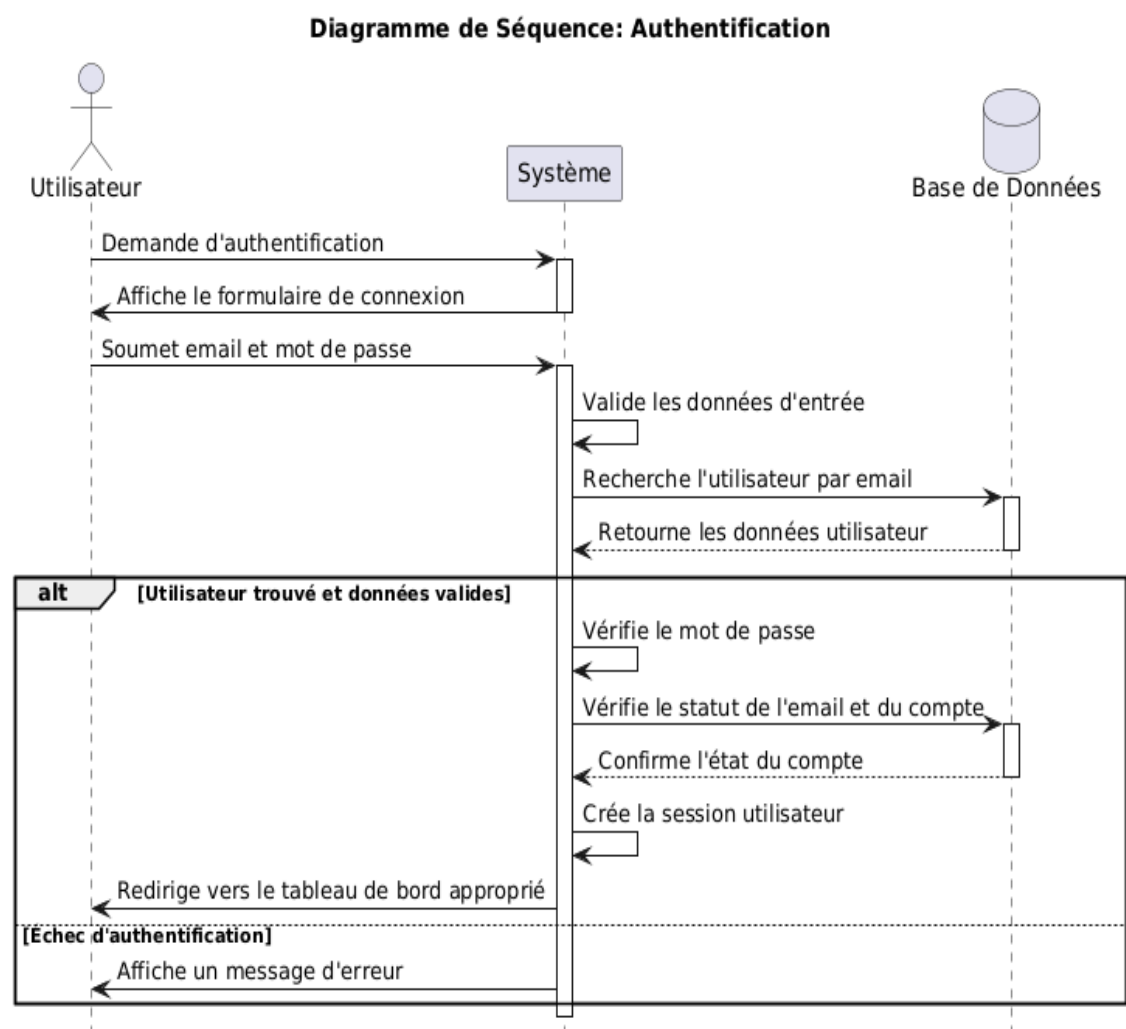
FIGURE 4.5 – Diagramme de séquence pour le scénario d'authentification
