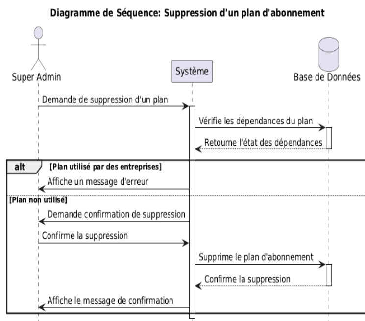
FIGURE 5.9 – Diagramme de séquence pour le scénario de suppression d'un plan d'abonnement
