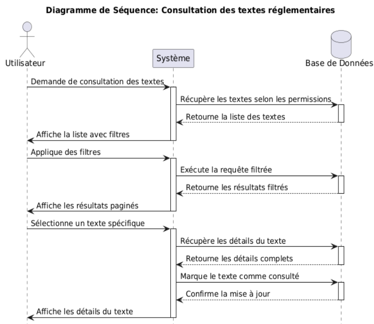
FIGURE 5.12 – Diagramme de séquence pour le scénario de consultation des textes réglementaires
