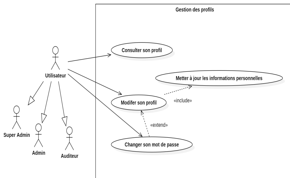
FIGURE 4.4 – Diagramme de cas d'utilisation - Gestion des profils
