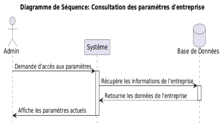
FIGURE 4.23 – Diagramme de séquence pour le scénario de consultation des paramètres d'entreprise
