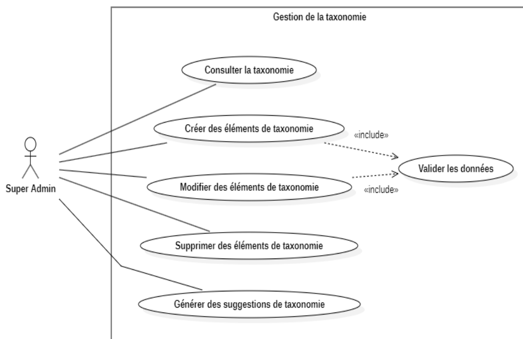
FIGURE 4.16 – Diagramme de cas d'utilisation - Gestion de la taxonomie
