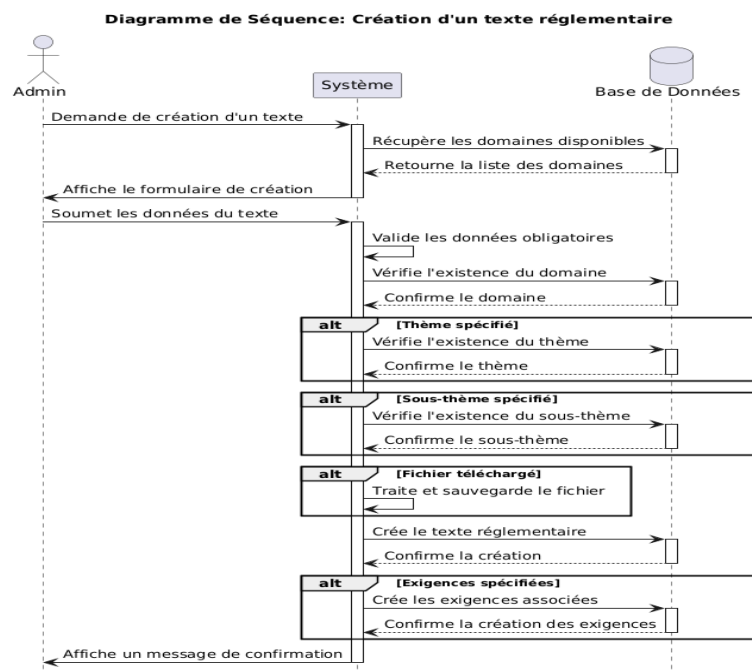
FIGURE 5.11 – Diagramme de séquence pour le scénario de création d'un texte réglementaire
