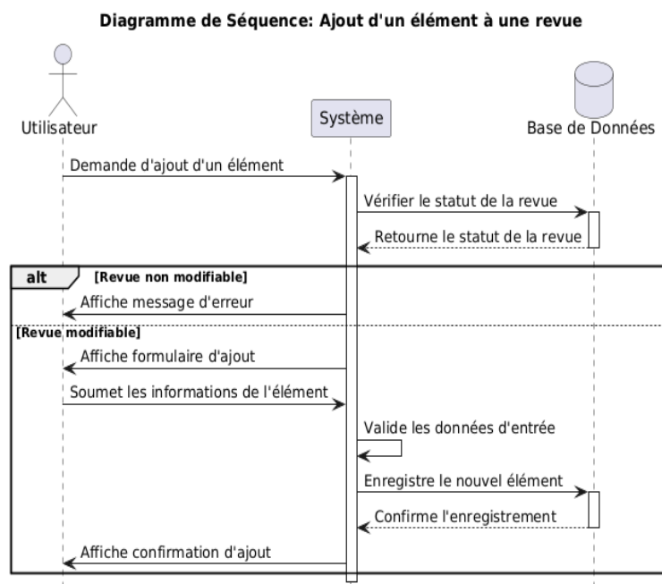
FIGURE 5.42 – Diagramme de séquence pour le scénario d'ajout d'un élément à une revue
