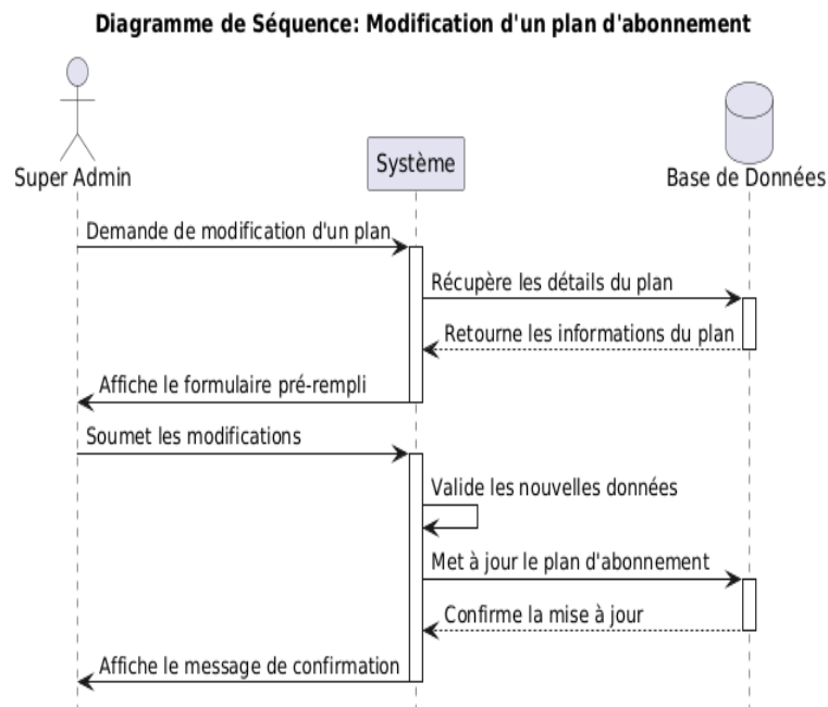
FIGURE 5.8 – Diagramme de séquence pour le scénario de modification d'un plan d'abonnement
