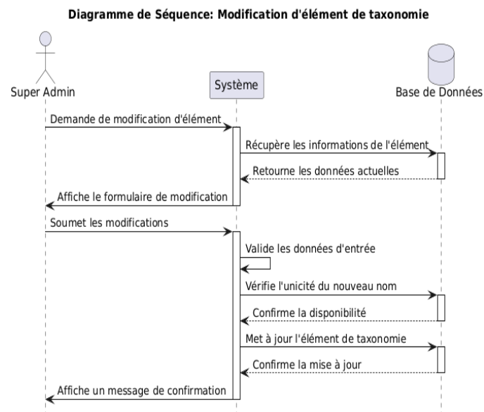
FIGURE 4.27 – Diagramme de séquence pour le scénario de modification d'élément de taxonomie
