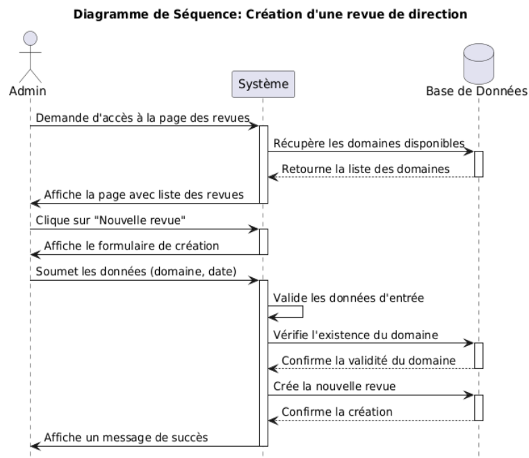
FIGURE 5.36 – Diagramme de séquence pour le scénario de création d'une revue de direction
