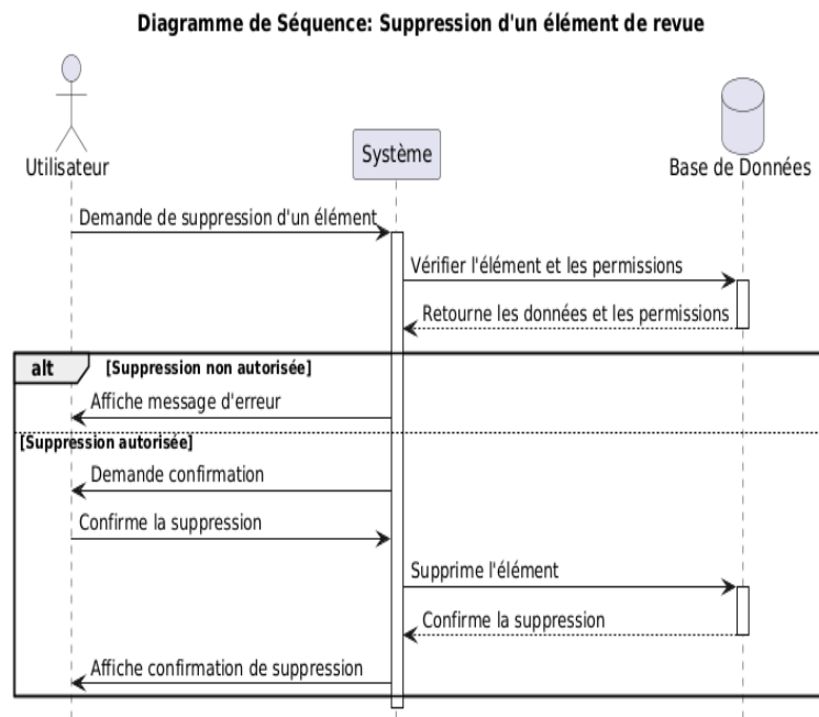
FIGURE 5.44 – Diagramme de séquence pour le scénario de suppression d'un élément de revue
