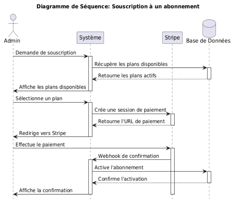
FIGURE 5.10 – Diagramme de séquence pour le scénario de souscription à un abonnement
