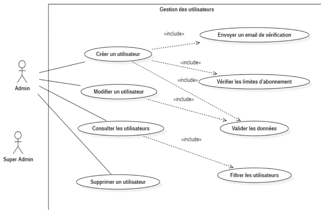
FIGURE 4.13 – Diagramme de cas d'utilisation - Gestion des utilisateurs
