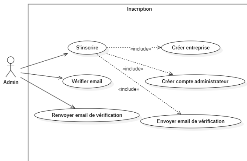
FIGURE 4.2 – Diagramme de cas d'utilisation - Inscription
