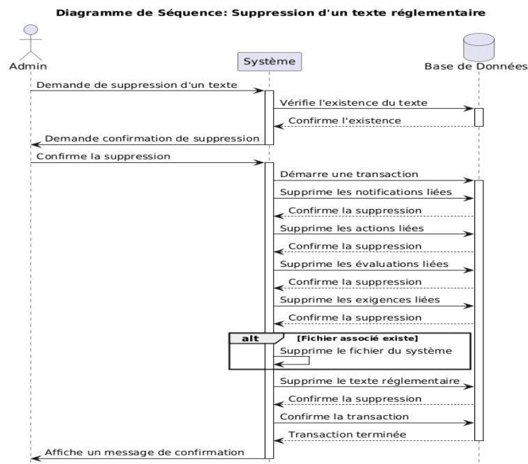
FIGURE 5.14 – Diagramme de séquence pour le scénario de suppression d'un texte réglementaire
