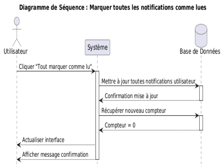
FIGURE 5.47 – Diagramme de séquence pour le scénario de marquage de toutes les notifications comme lues
