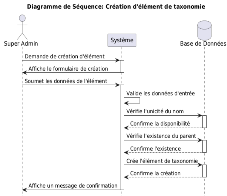
FIGURE 4.25 – Diagramme de séquence pour le scénario de création d'élément de taxonomie
