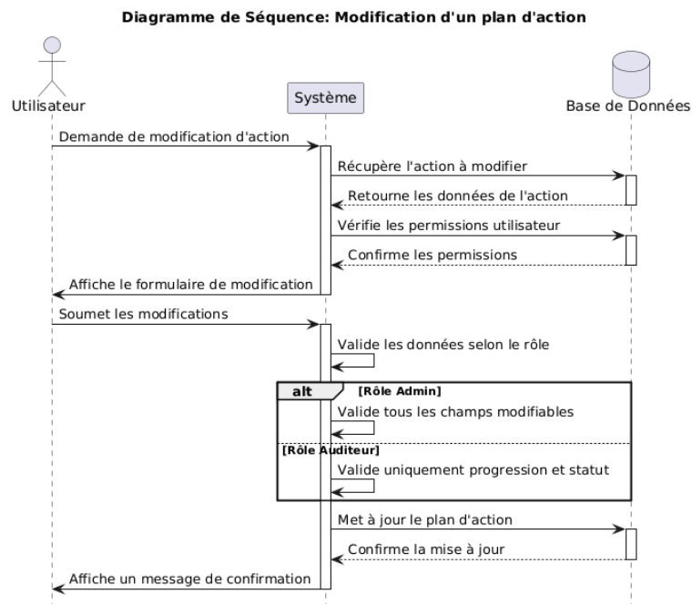
FIGURE 5.18 – Diagramme de séquence pour le scénario de modification d'un plan d'action
