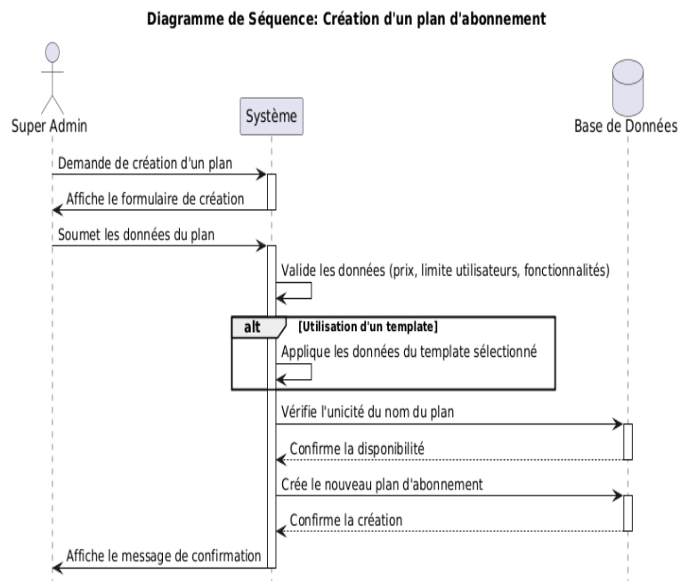
FIGURE 5.6 – Diagramme de séquence pour le scénario de création d'un plan d'abonnement
