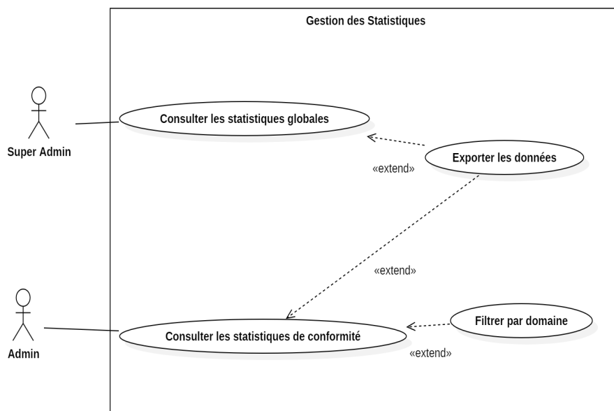
FIGURE 5.35 – Diagramme de cas d'utilisation - Consultation des statistiques
