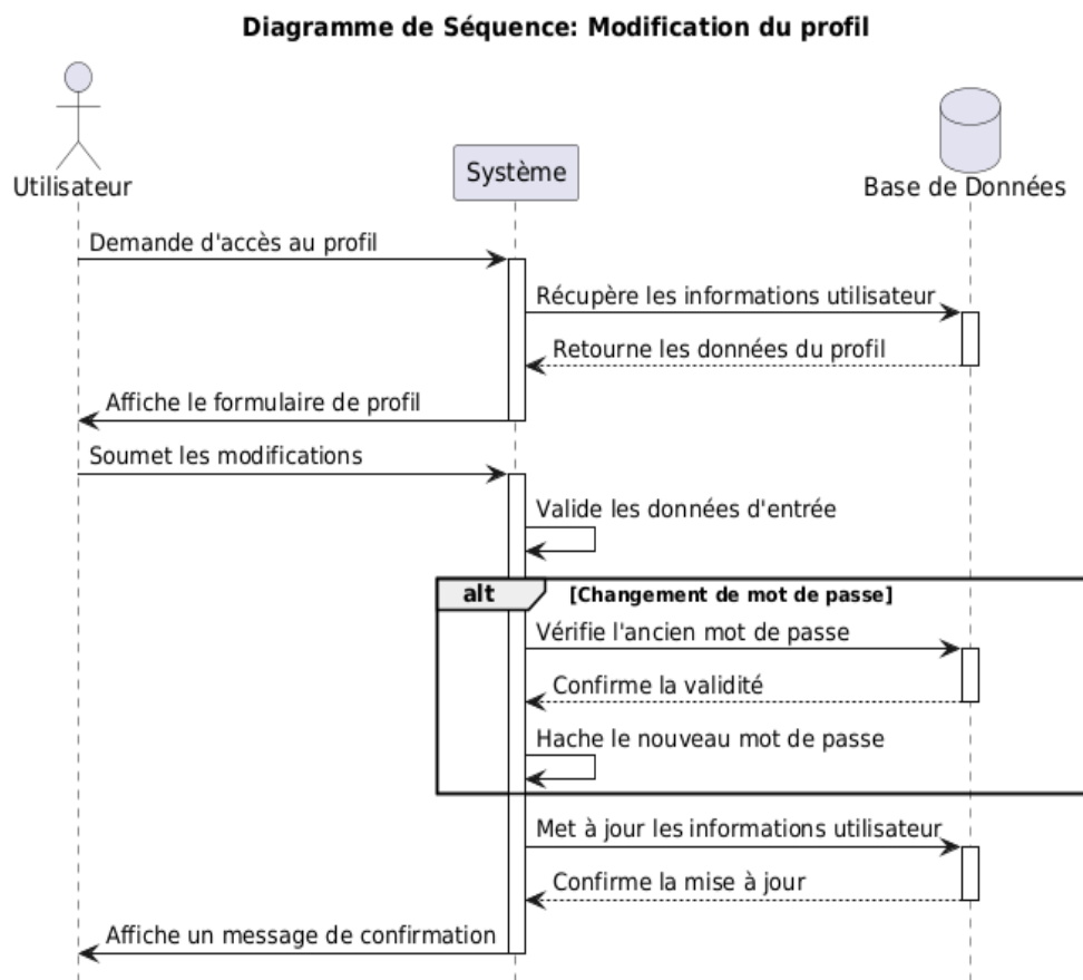
FIGURE 4.8 – Diagramme de séquence pour le scénario de modification du profil
