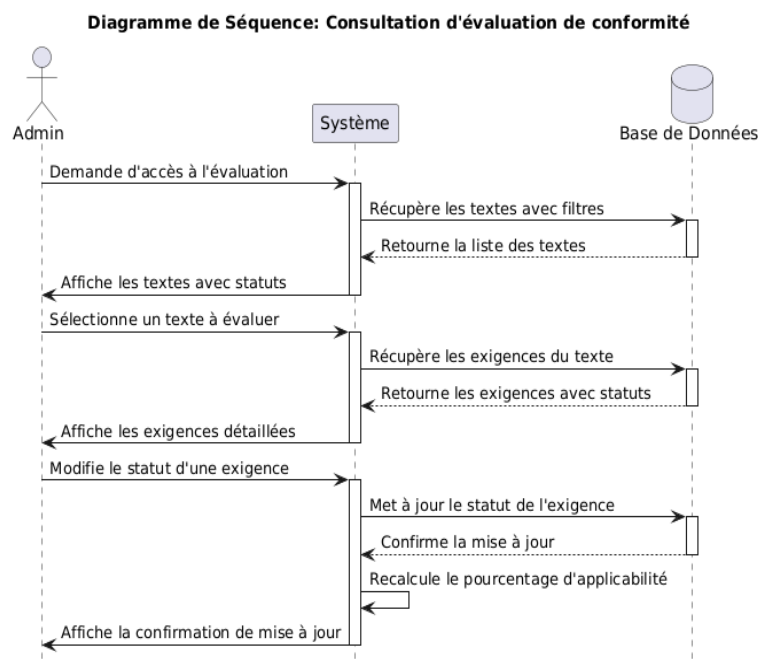
FIGURE 5.15 – Diagramme de séquence pour le scénario d'évaluation de conformité
