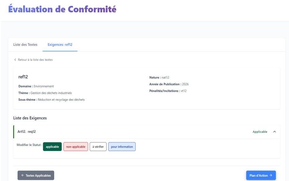
FIGURE 5.27 – Interface d’évaluation des exigences
