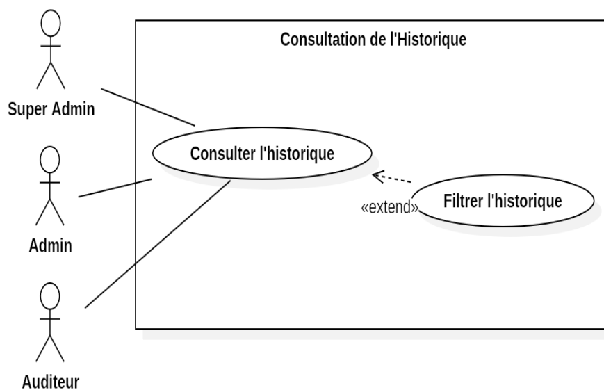
FIGURE 5.34 – Diagramme de cas d'utilisation - Consultation de l'historique
