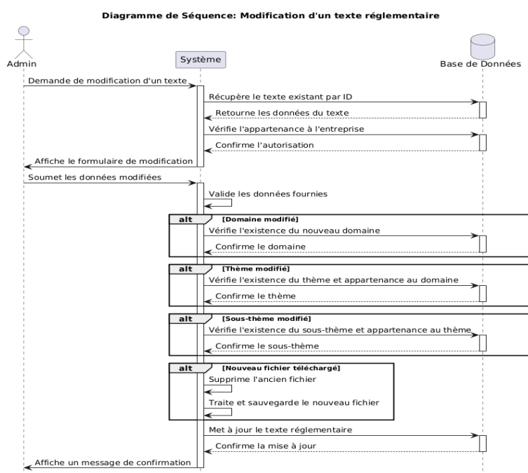
FIGURE 5.13 – Diagramme de séquence pour le scénario de modification d'un texte réglementaire
