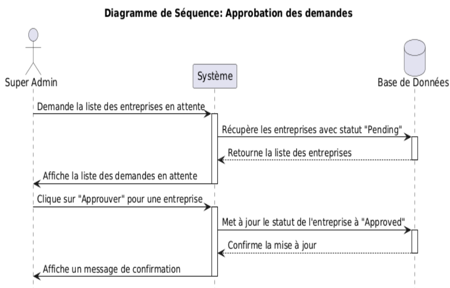
FIGURE 4.7 – Diagramme de séquence pour le scénario d'approbation des demandes
