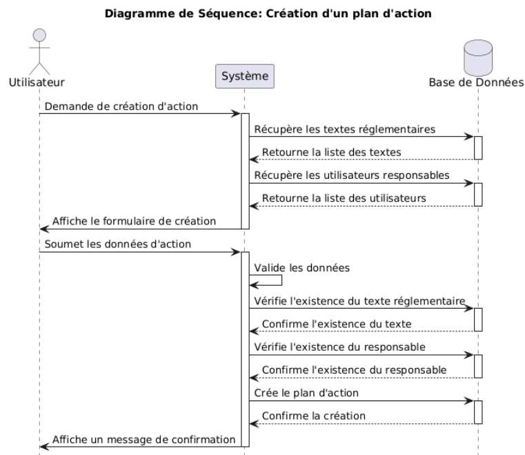
FIGURE 5.16 – Diagramme de séquence pour le scénario de création d'un plan d'action
