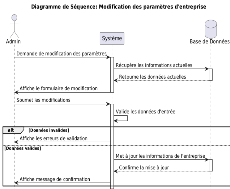
FIGURE 4.24 – Diagramme de séquence pour le scénario de modification des paramètres d'entreprise
