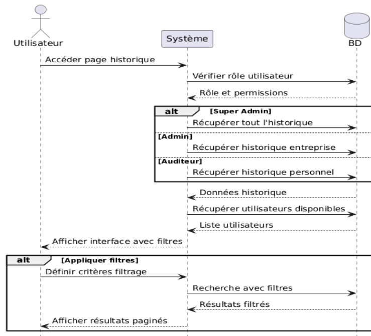
FIGURE 5.48 – Diagramme de séquence pour le scénario de consultation de l'historique
