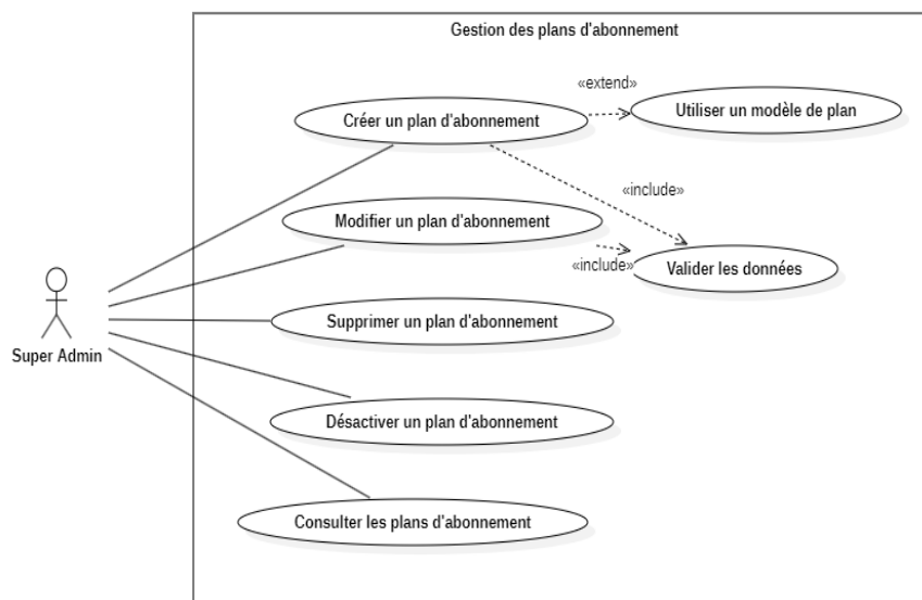
FIGURE 5.1 – Diagramme de cas d'utilisation - Gestion des plans d'abonnement
