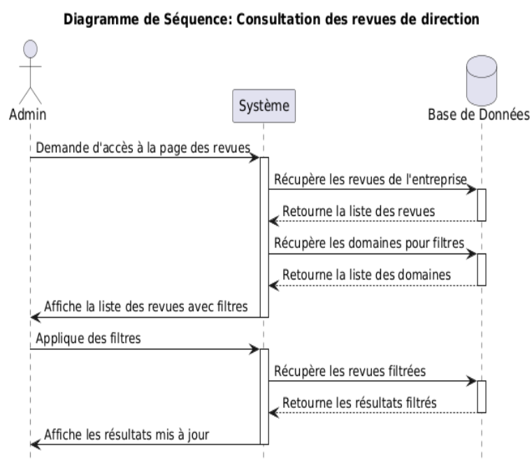
FIGURE 5.37 – Diagramme de séquence pour le scénario de consultation des revues de direction
