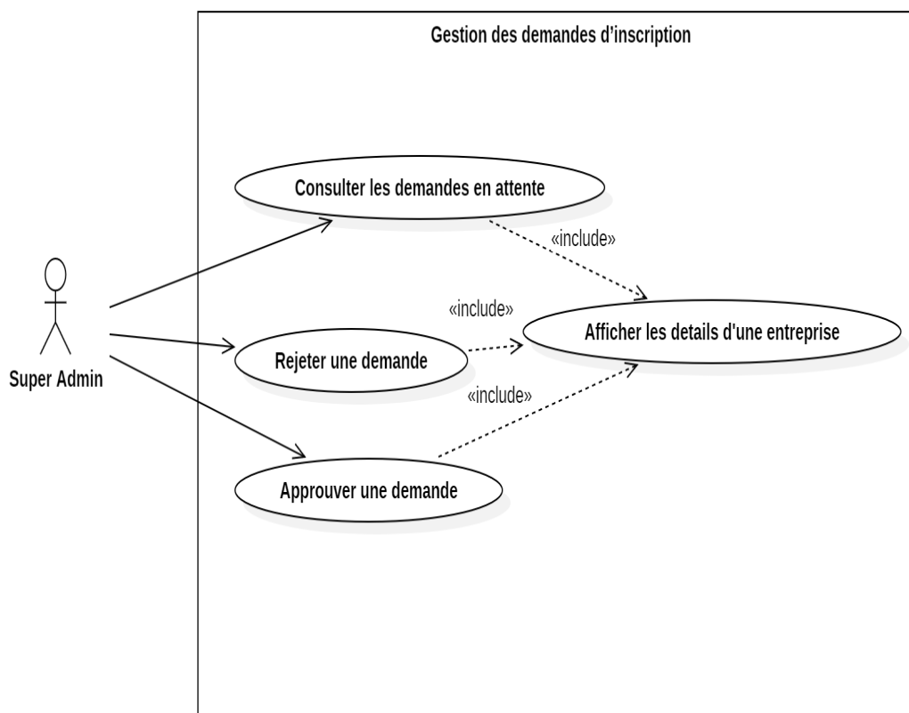
FIGURE 4.3 – Diagramme de cas d'utilisation - Gestion des demandes d'inscription
