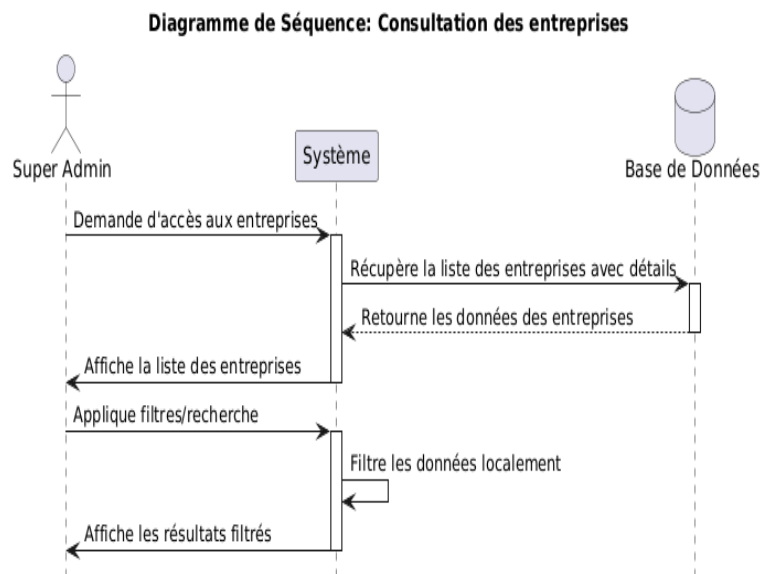
FIGURE 4.21 – Diagramme de séquence pour le scénario de consultation des entreprises
