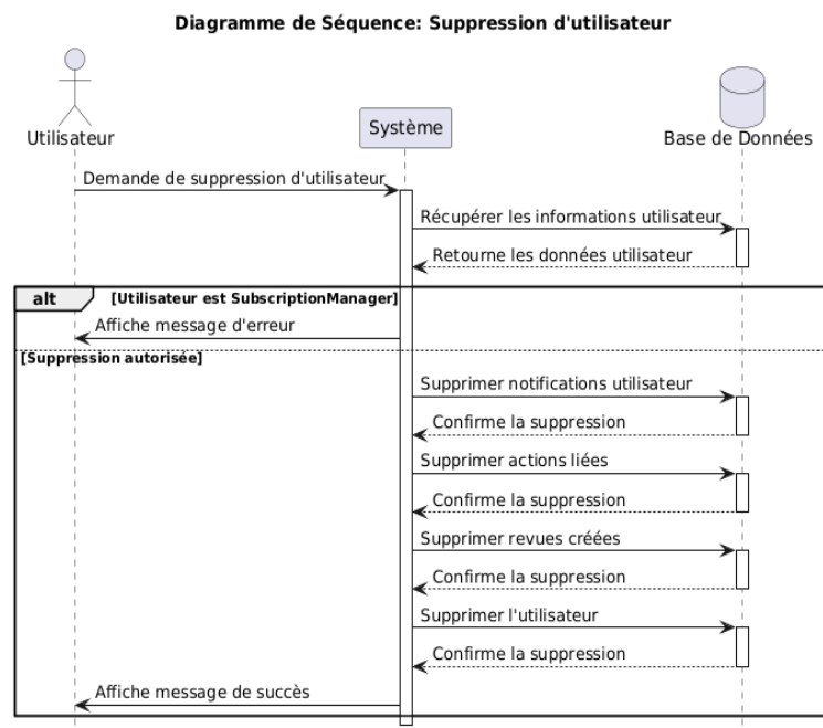
FIGURE 4.20 – Diagramme de séquence pour le scénario de suppression d'utilisateur
