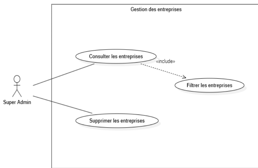
FIGURE 4.14 – Diagramme de cas d'utilisation - Gestion des entreprises
