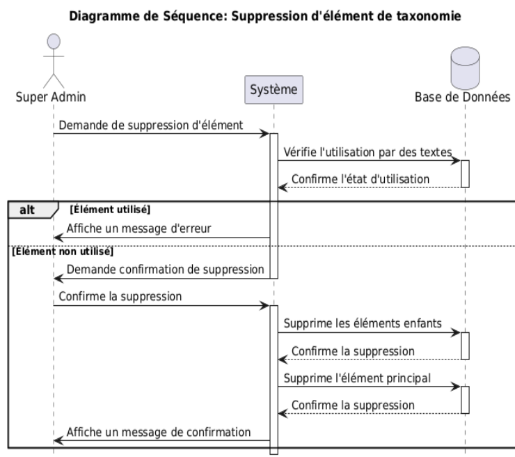
FIGURE 4.28 – Diagramme de séquence pour le scénario de suppression d'élément de taxonomie
