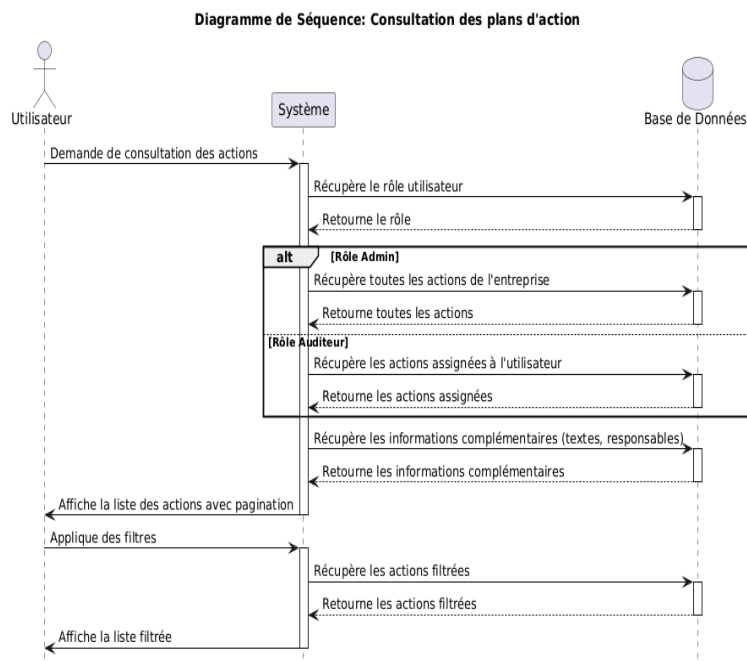
FIGURE 5.17 – Diagramme de séquence pour le scénario de consultation des plans d'action
