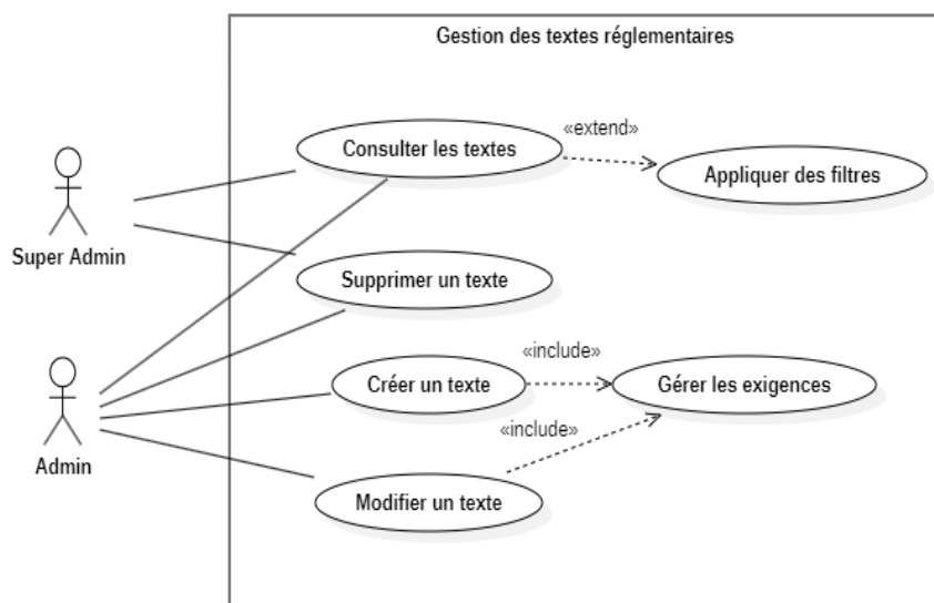
FIGURE 5.3 – Diagramme de cas d'utilisation - Gestion des textes réglementaires
