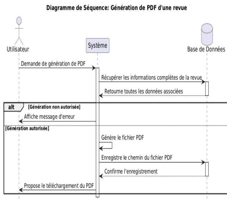
FIGURE 5.45 – Diagramme de séquence pour le scénario de génération de PDF d'une revue
