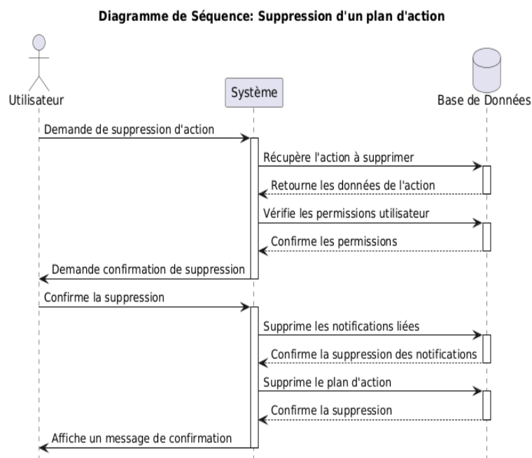
FIGURE 5.19 – Diagramme de séquence pour le scénario de suppression d'un plan d'action
