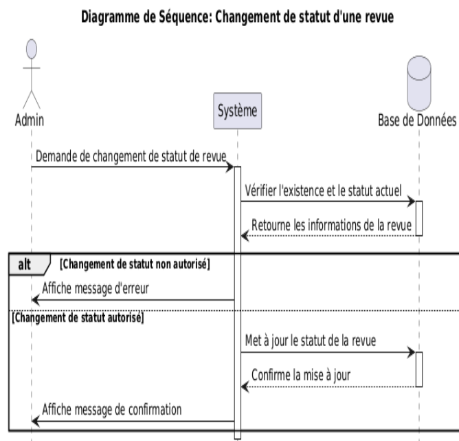
FIGURE 5.40 – Diagramme de séquence pour le scénario de changement de statut d'une revue
