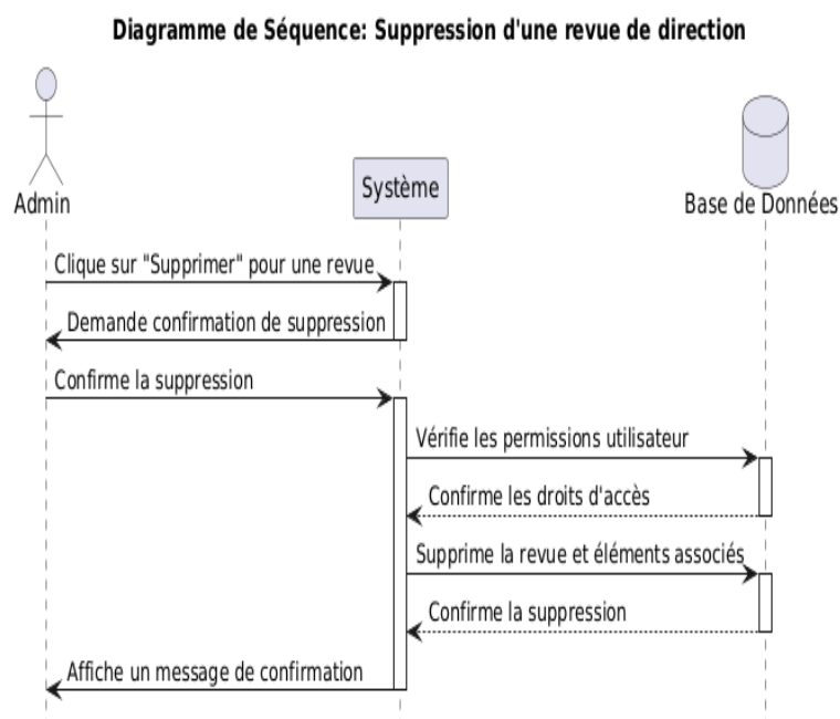
FIGURE 5.39 – Diagramme de séquence pour le scénario de suppression d'une revue de direction
