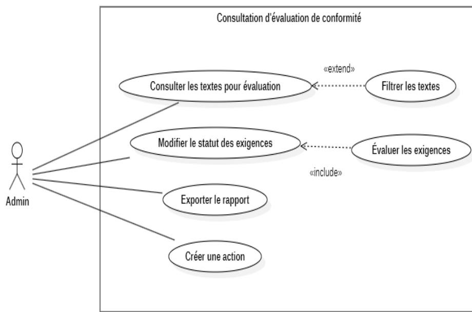
FIGURE 5.4 – Diagramme de cas d'utilisation - Évaluation de conformité
