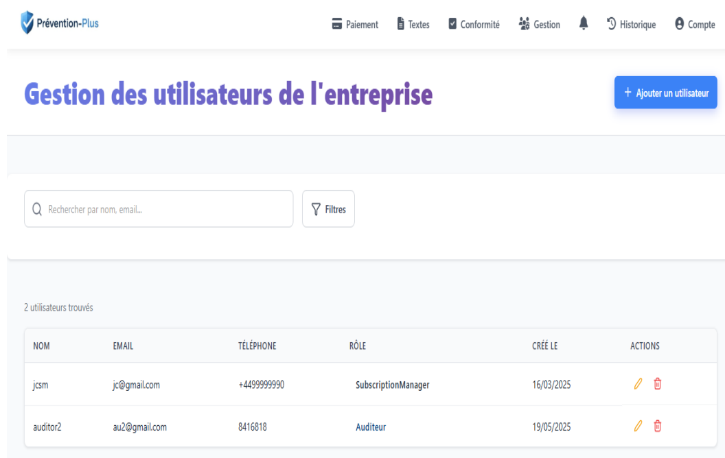
FIGURE 4.30 – Interface de gestion des utilisateurs - Admin
