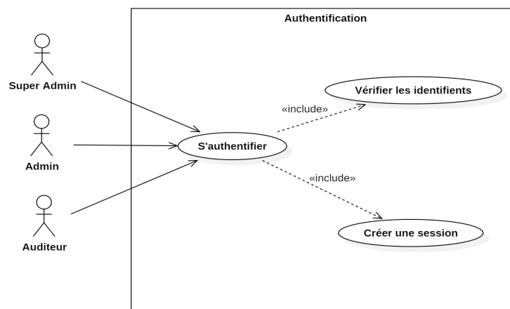
FIGURE 4.1 – Diagramme de cas d'utilisation - Authentification
